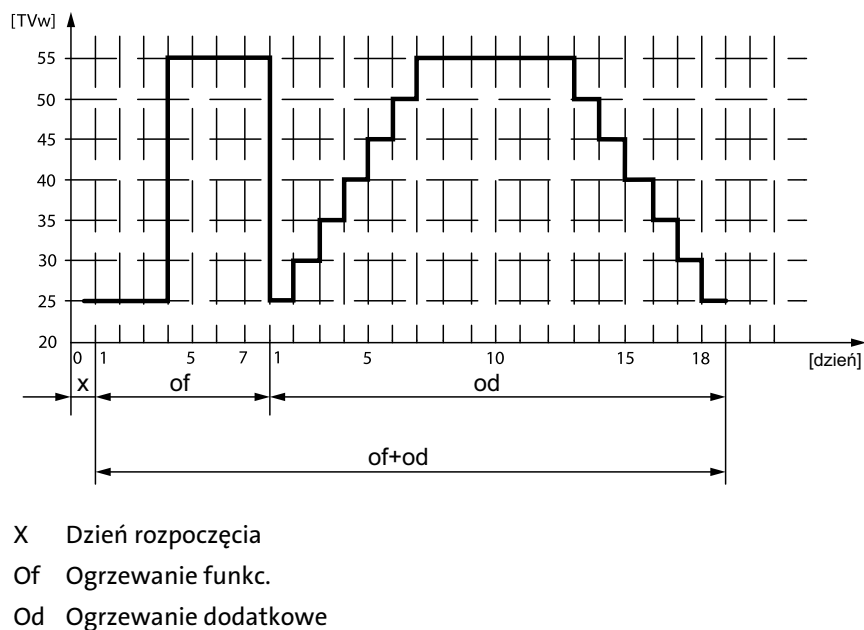
Rys. 23: Profil temperatury dla funkcji osuszania jastrychu
