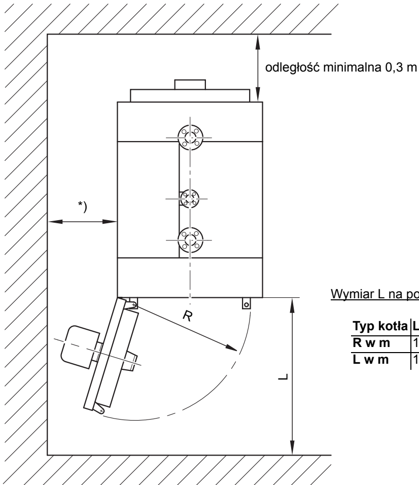
Rys. 3: Zapotrzebowanie na miejsce kotłów serii LogoBloc L 400-600 C
