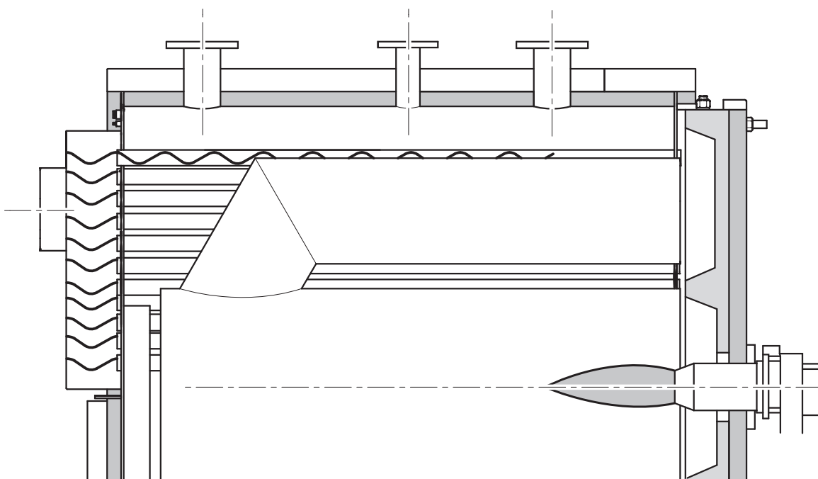
Rys. 2: Prawidłowe położenie turbolizatorów
