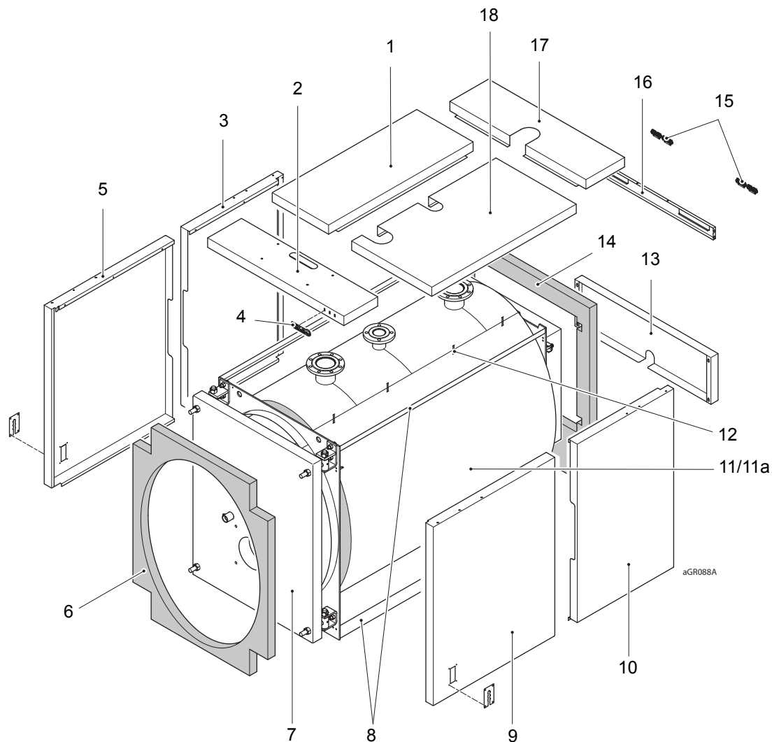
Rys. 5: Montaż
