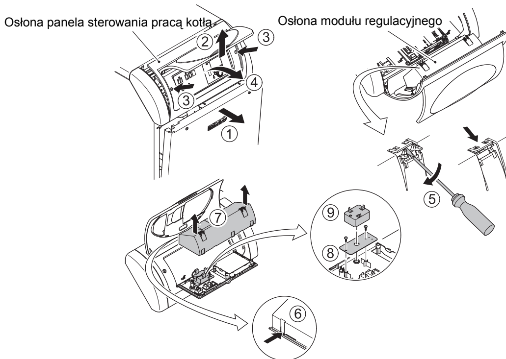
Rys. 11: Odblokowanie ogranicznika temperatury bezpieczeństwa STB
