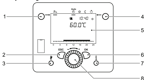
Rys. 9: Elementy obsługi
