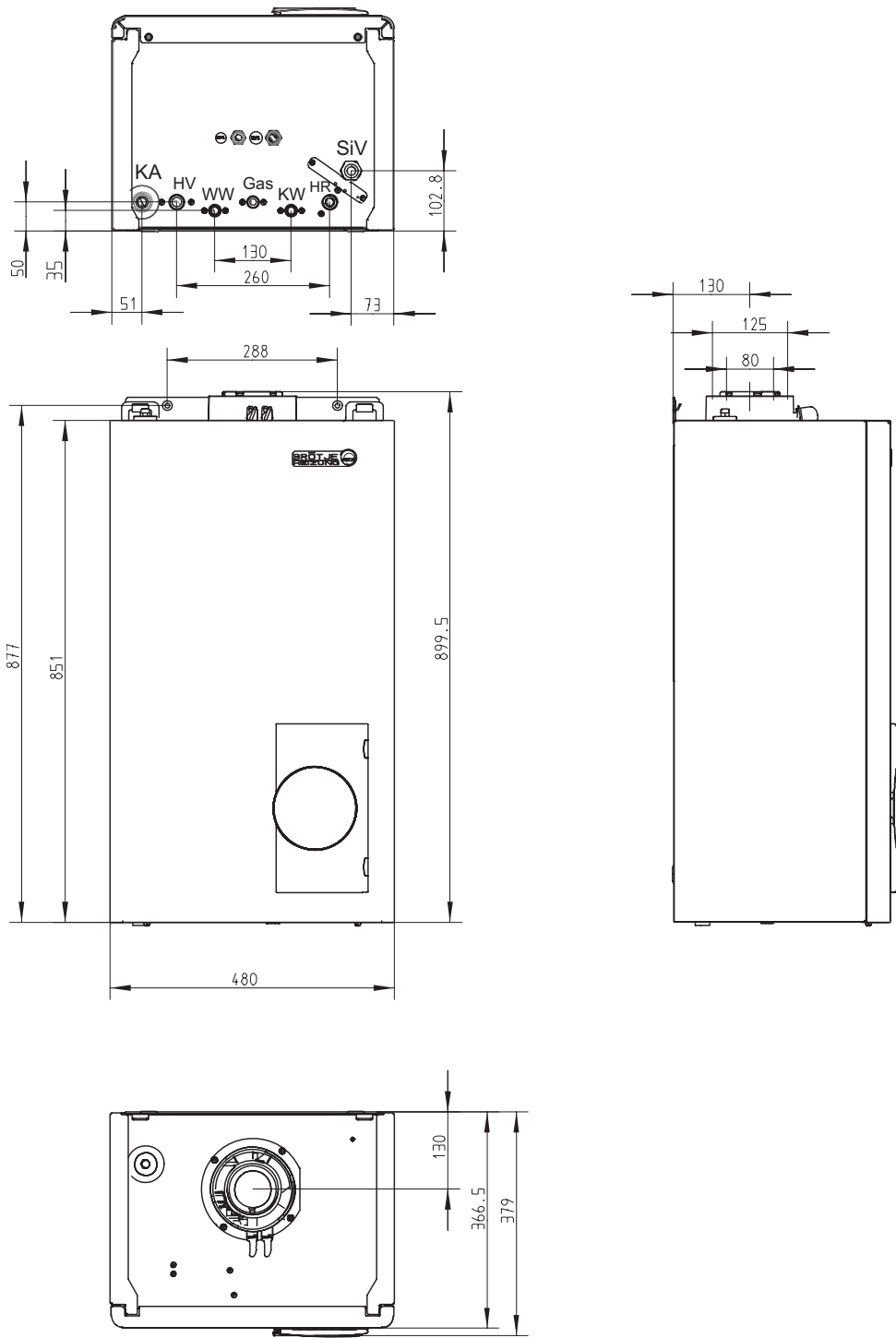
Rys. 1: Wymiary i przyłącza
