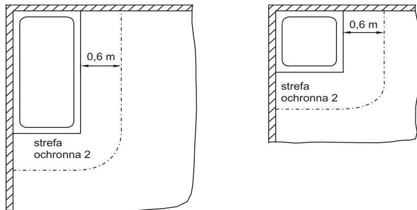
Rys. 3: Odległości od kotła WBC w łazienkach i pomieszczeniach z natryskami
