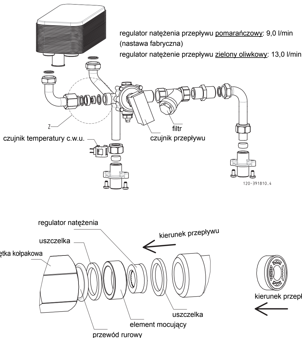
Rys. 4: Wymiana regulatora natężenia przepływu
