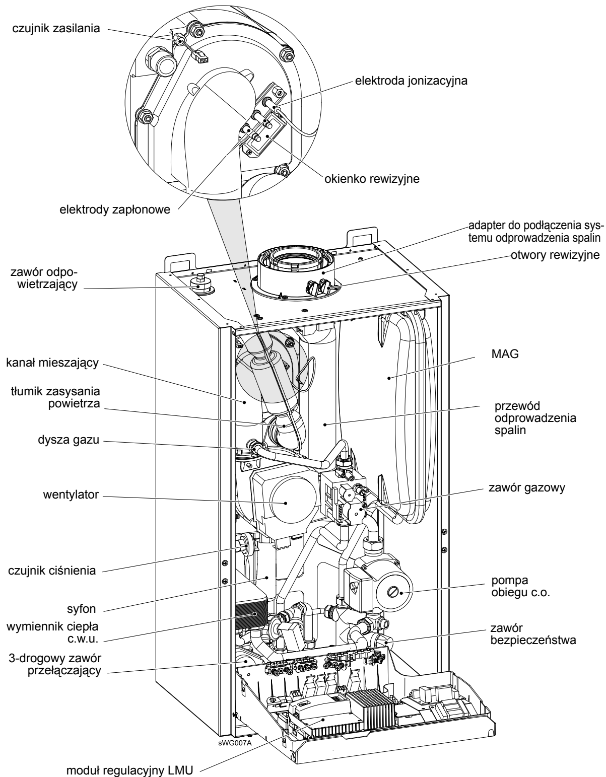
Rys. 20: Widok kotła WBC (na rysunku bez ścianki przedniej i pokrywy zespołu regulacyjnego)
