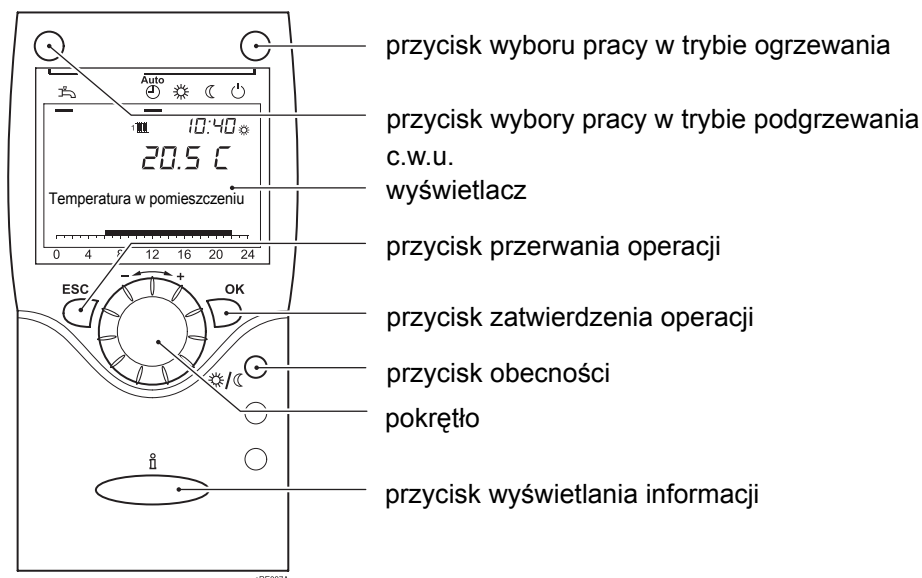
Rys. 21: Panel obsługowy regulatorów RGT
