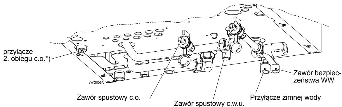
Rys. 4: Strona dolna kotła WBK
