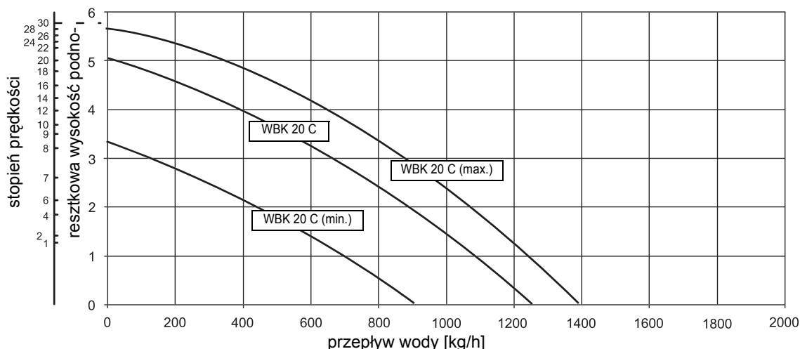
Rys. 16: Resztkowa wysokość podnoszenia
