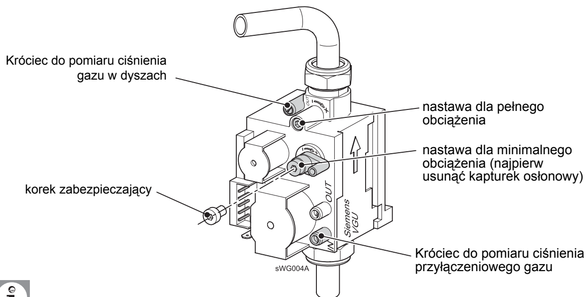
Rys. 9: Armatura gazowa (nastawa ciśnienia dyszy za pomocą klucza Torx T15)
