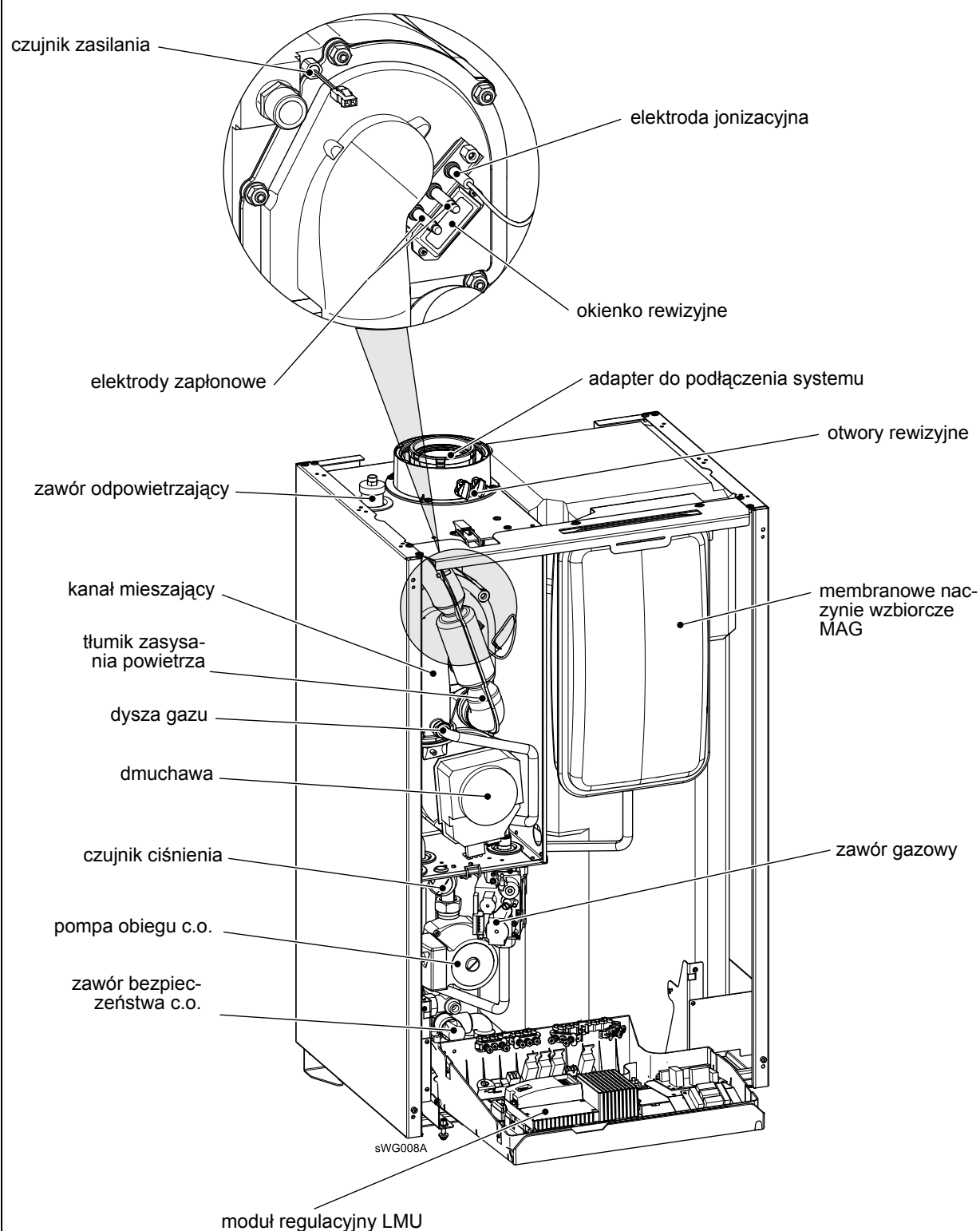
Rys. 23: Widok kotła WBK (na rysunku bez ścianki przedniej i pokrywy zespołu regulacyjnego)
