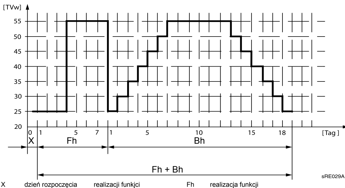
Rys. 15: Profil temperatury dla funkcji osuszania jastrychu
