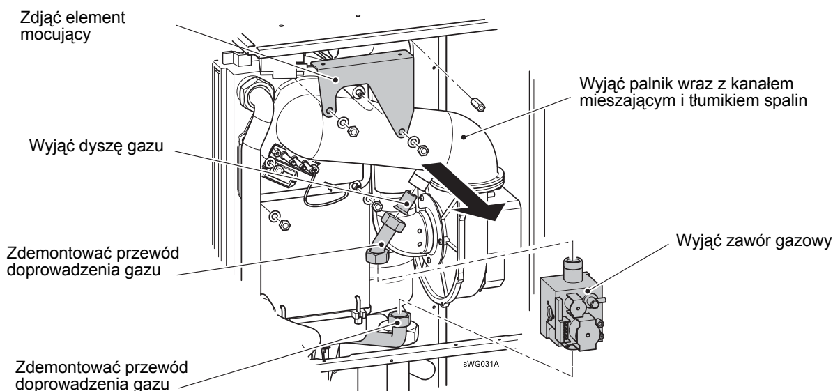
Rys. 20: Wymontować palnik gazowy (kocioł WGB 50 D)
