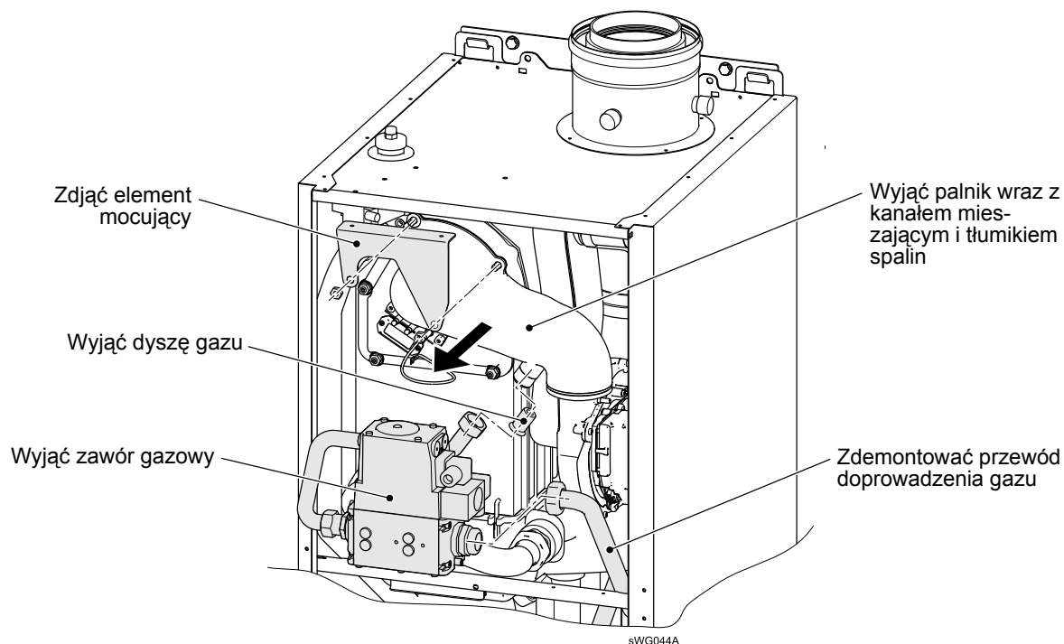
Rys. 22: Wymontować palnik gazowy (kocioł WGB 90/110 C)
