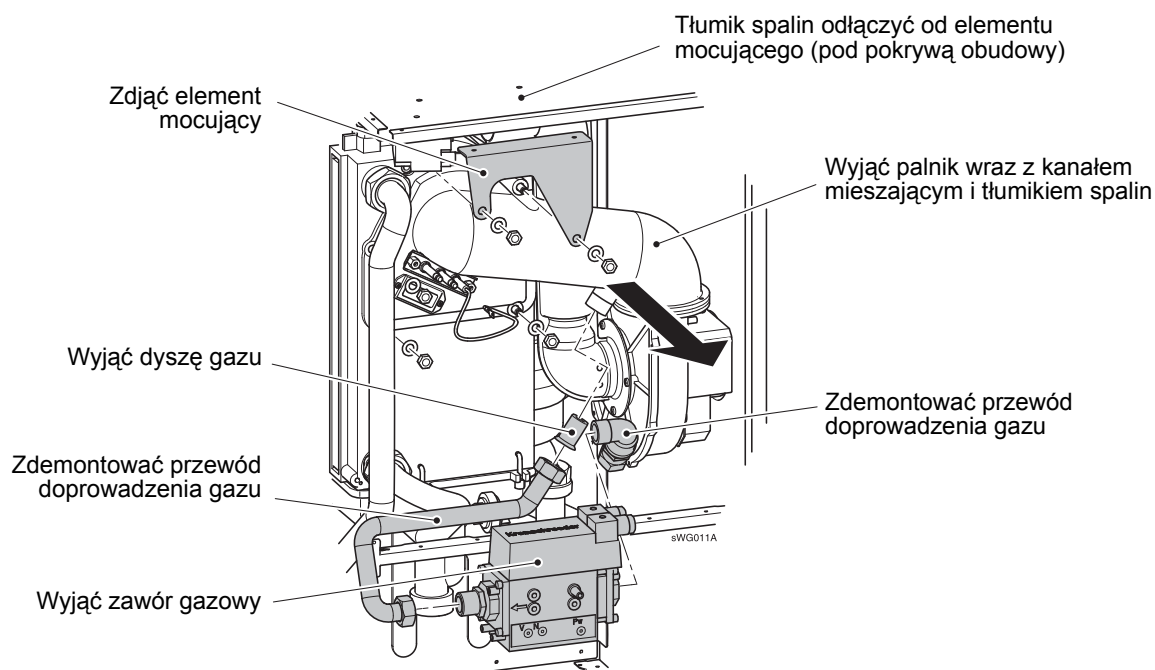
Rys. 21: Wymontować palnik gazowy (kocioł WGB 70 D)
