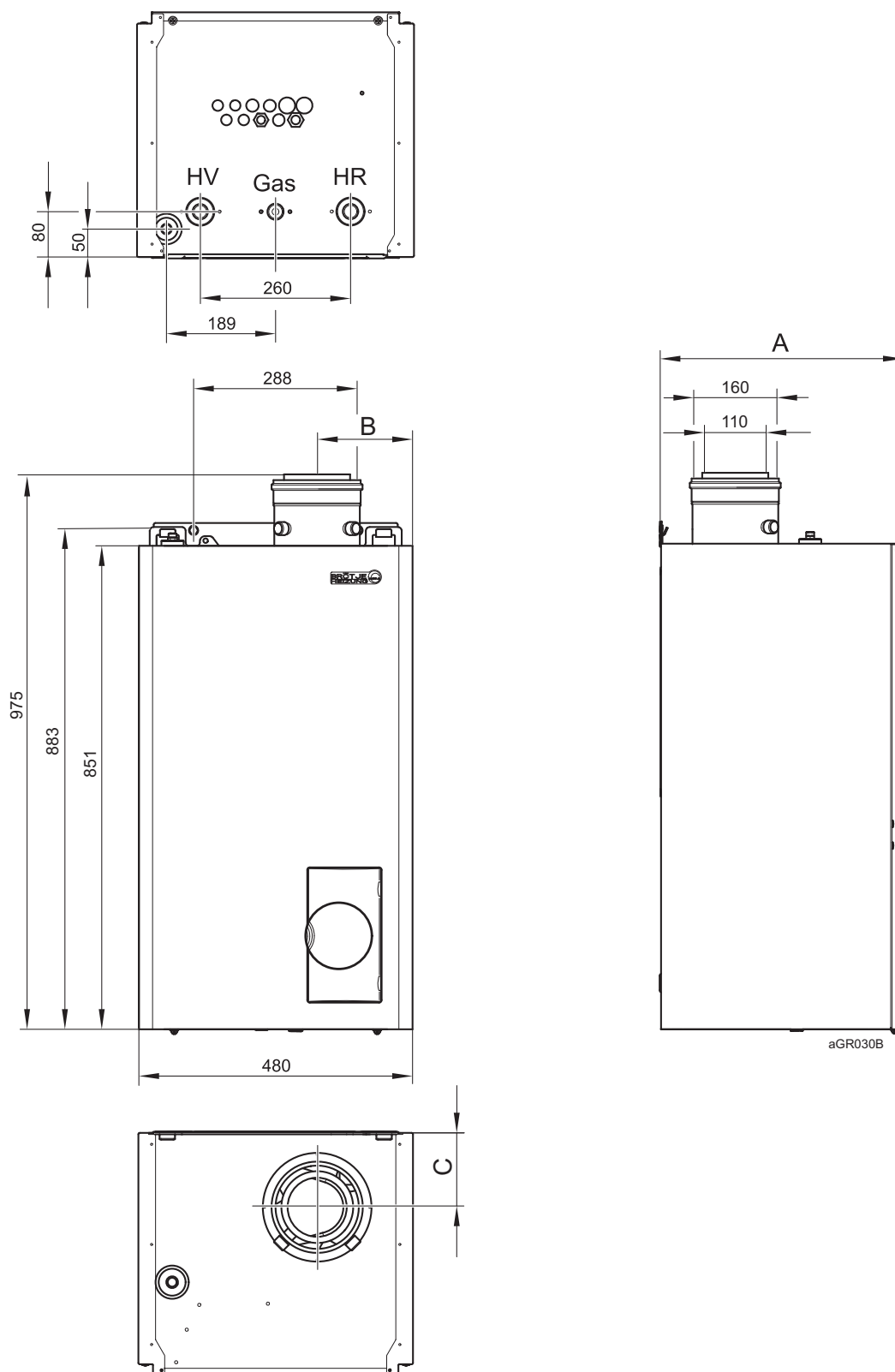
Rys. 1: Wymiary i przyłącza
