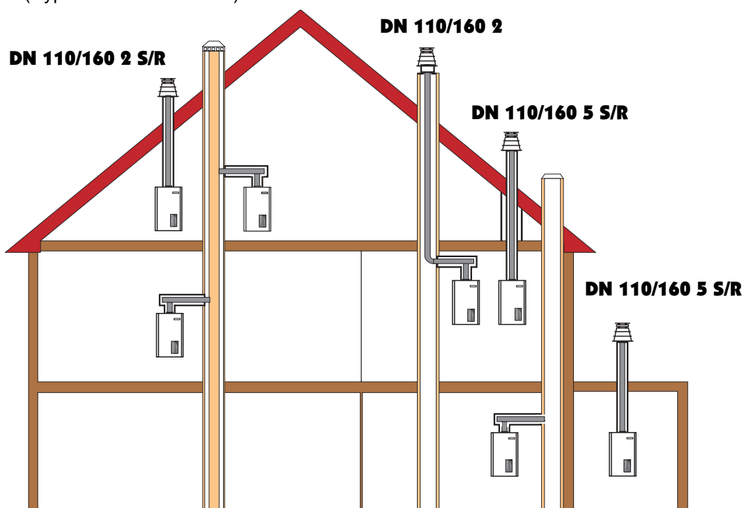
Rys. 4: Możliwości zamontowania kotła z zastosowaniem systemu odprowadzenia spalin (wyposażenie dodatkowe)
