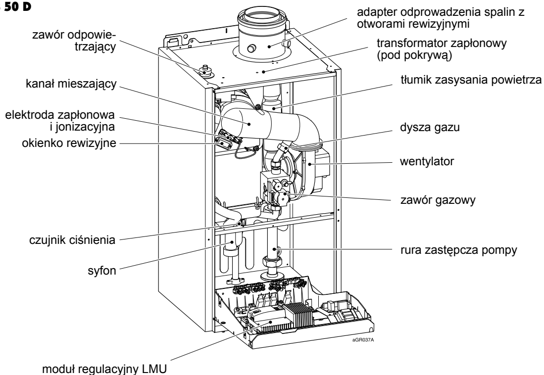
Rys. 23: Widok kotła (na rysunku bez przedniej ścianki obudowy i pokrywy zespołu regulacyjnego)
