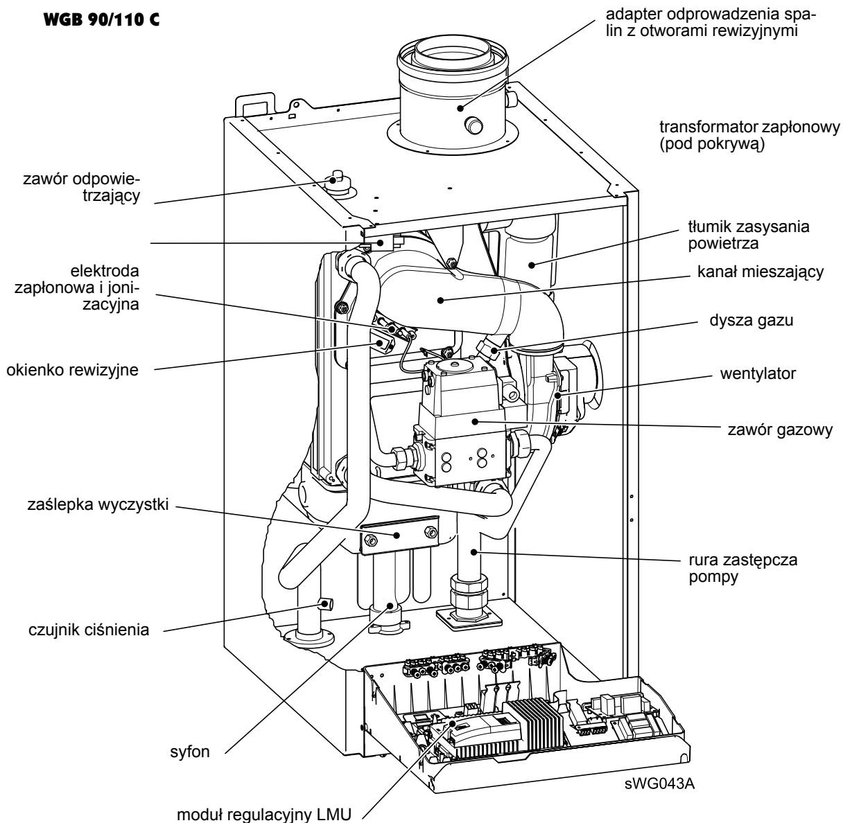
Rys. 24: Widok kotła (na rysunku bez przedniej ścianki obudowy i pokrywy zespołu regulacyjnego)
