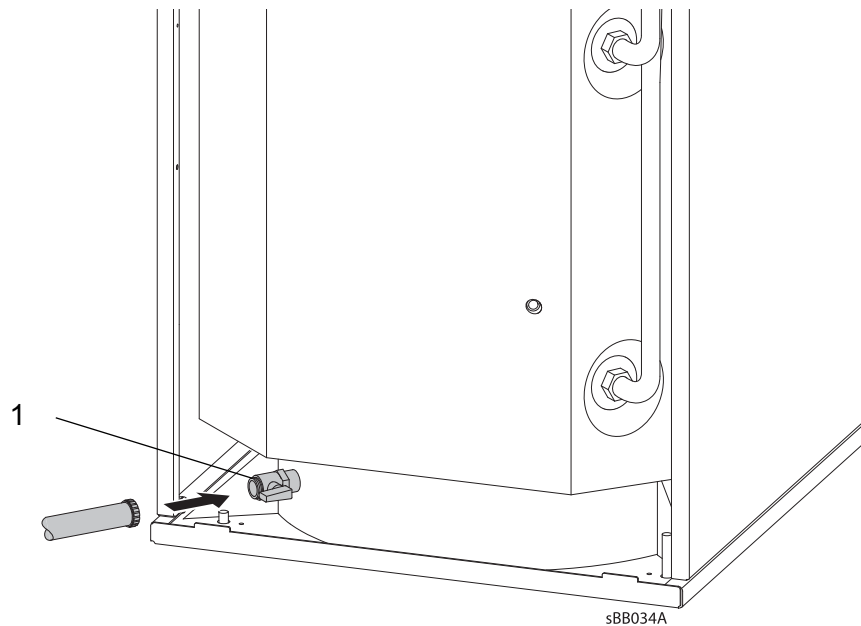
Rys. 17: Spuszczanie wody z podgrzewacza c.w.u. (podgrzewacz RSP z węzownicą)
