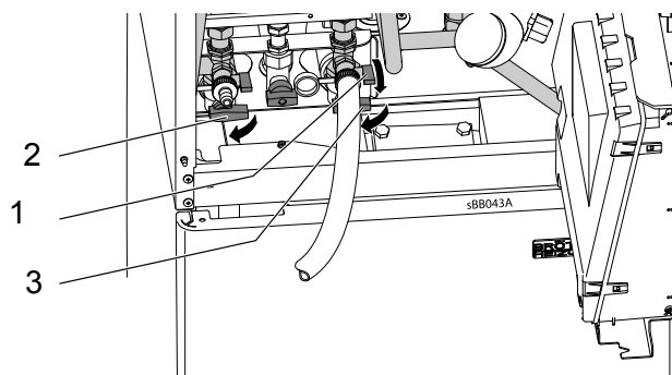
Rys. 11: Napełnianie instalacji c.o. (podgrzewacz RSP z wężownicą)
