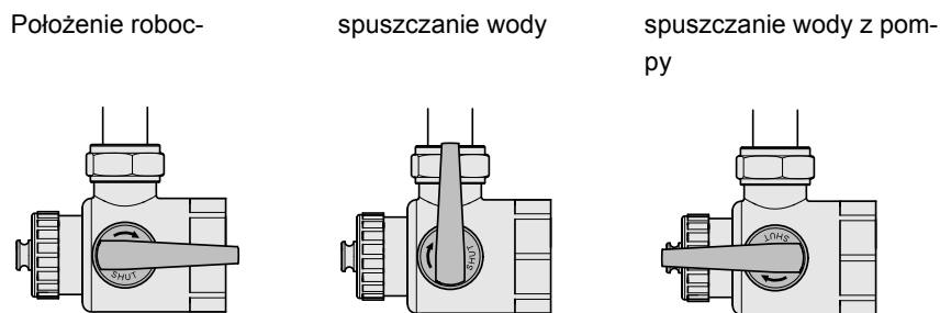
Rys. 18: Położenia zaworu spustowego podgrzewacza c.w.u. (tylko podgrzewacz warstwowy SSP)
