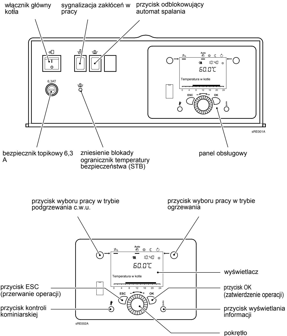
Rys. 1: Elementy obsługi
