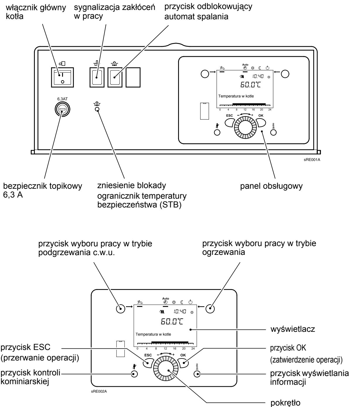
Rys. 1: Elementy obsługi
