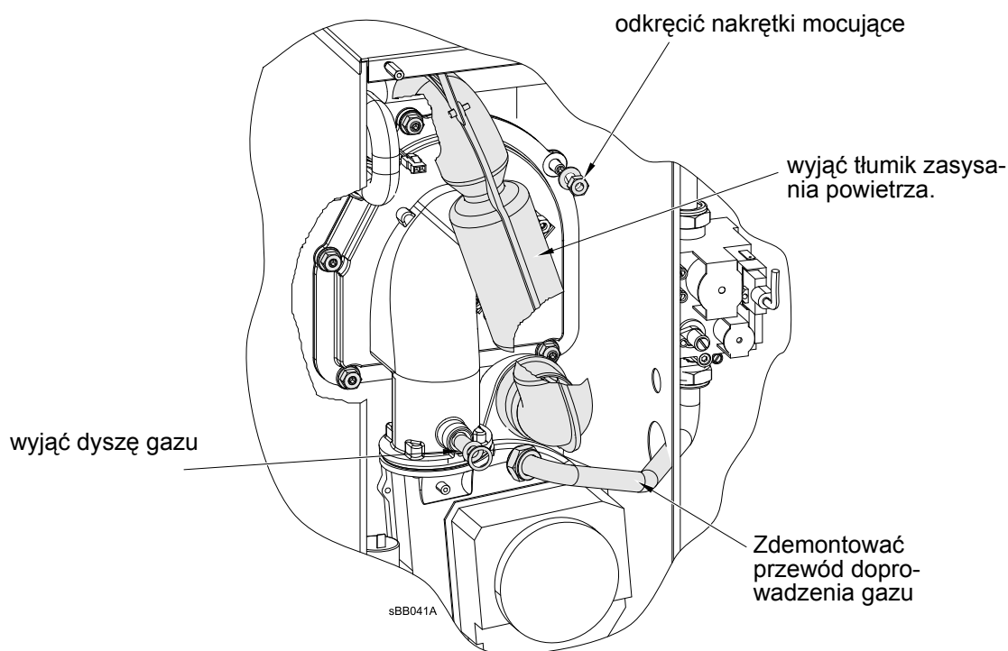
Rys. 20: Wymontowywanie palnika gazowego
