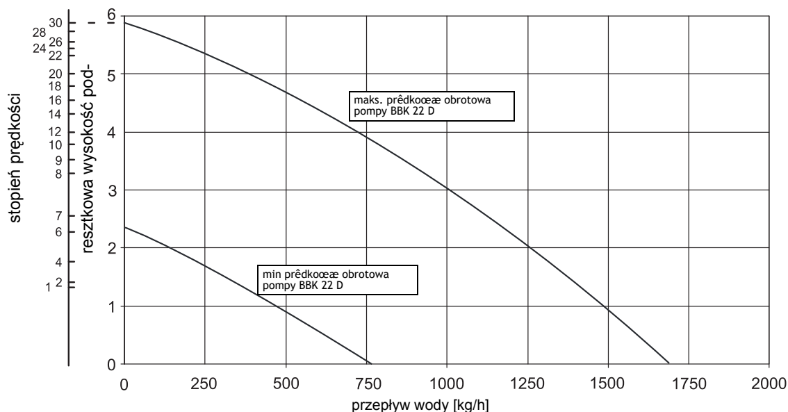
Rys. 16: Resztkowa wysokość podnoszenia
