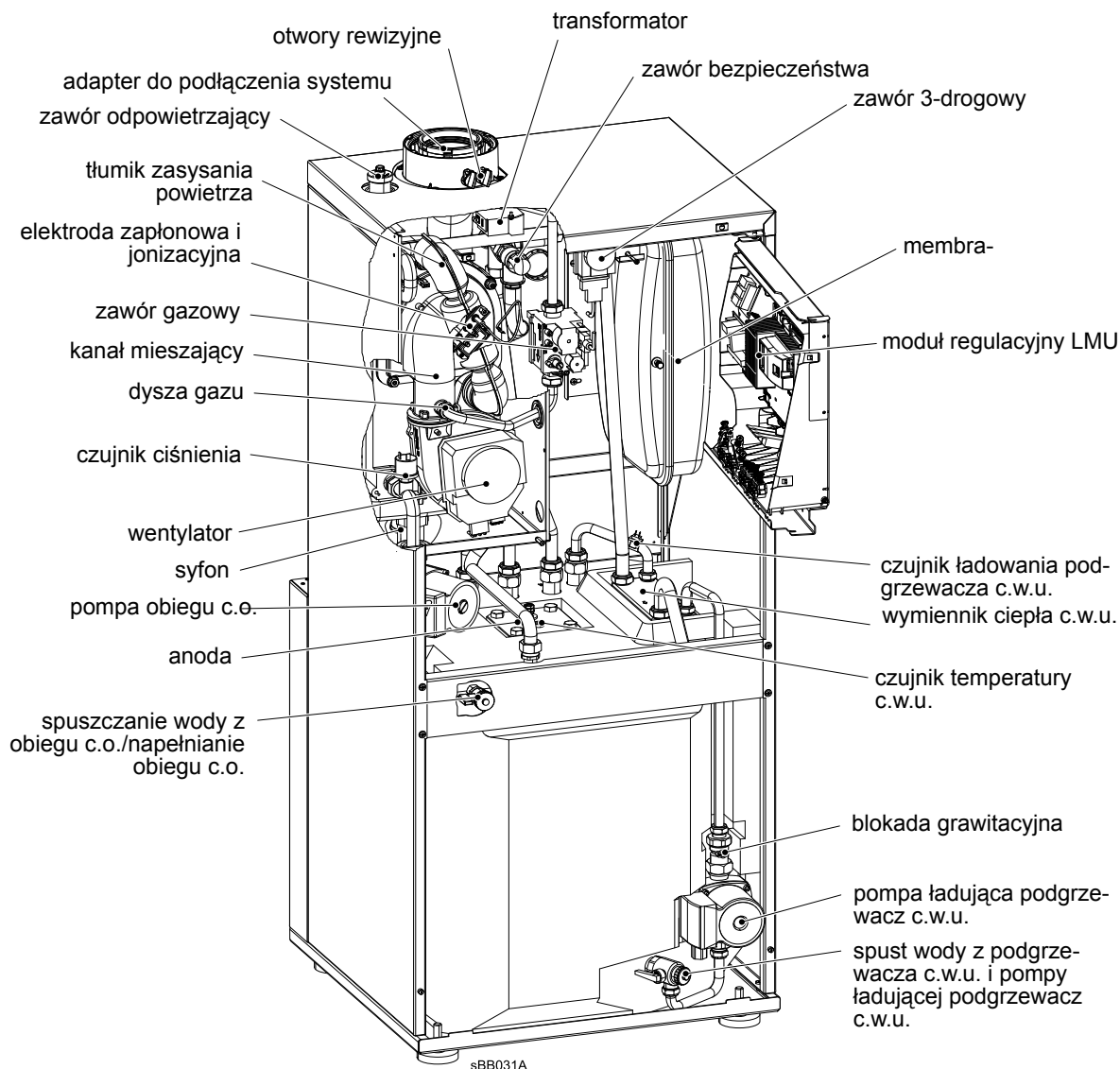
Rys. 21: Widok kotła BBK (na rysunku bez ścianki przedniej i pokrywy zespołu regulacyjnego)
