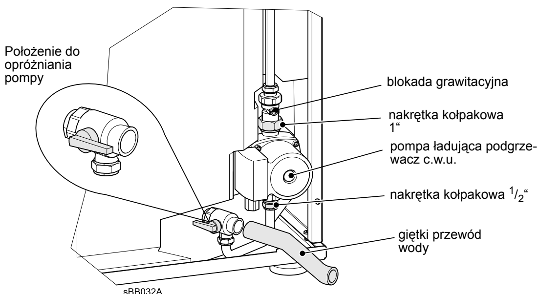
Rys. 24: Demontaż pompy ładującej podgrzewacz c.w.u.
