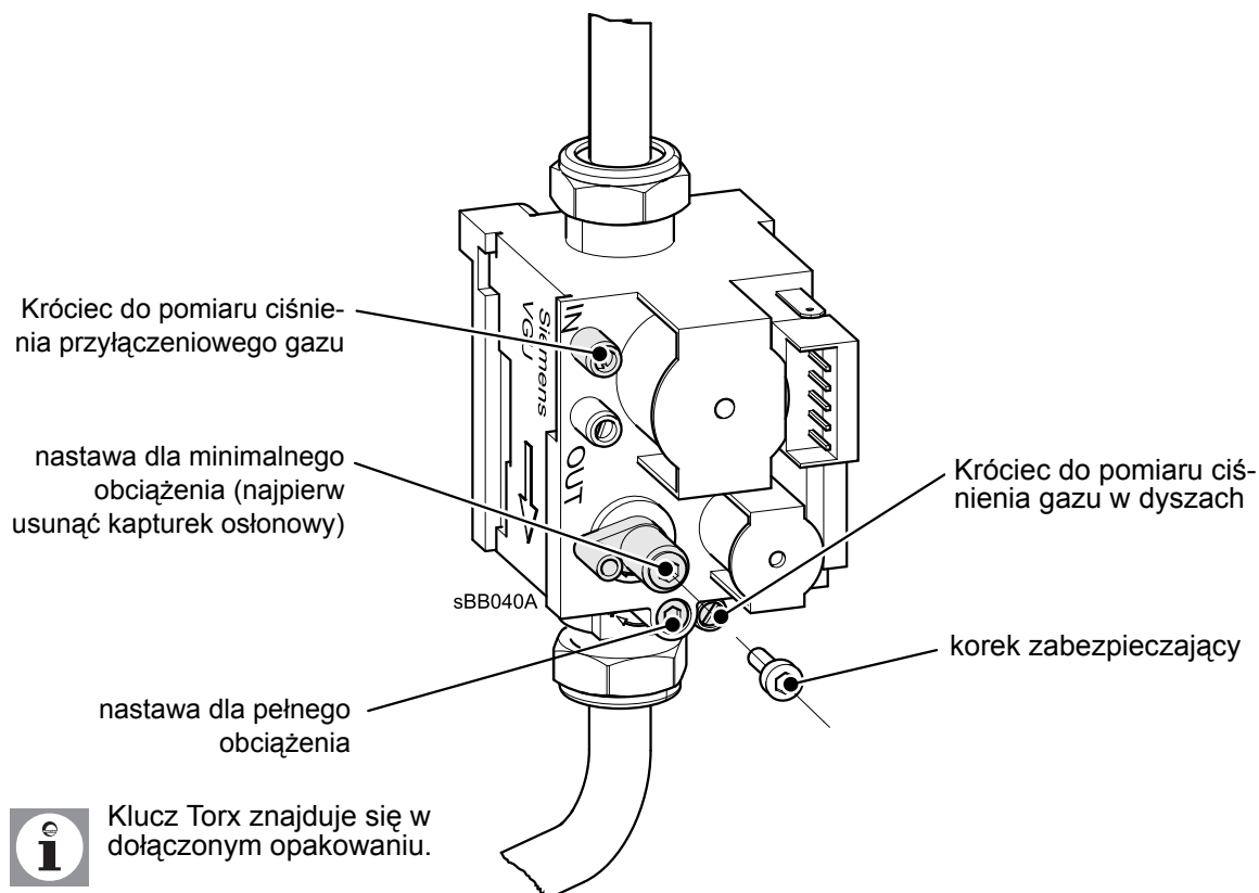
Rys. 9: Armatura gazowa (nastawa ciśnienia dyszy za pomocą klucza Torx T15)
