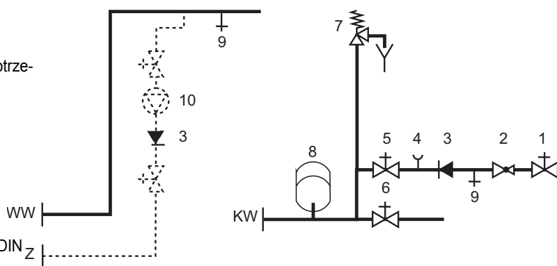
Rys. 4: Przykład montażu zgodnie z normą DIN 1988
