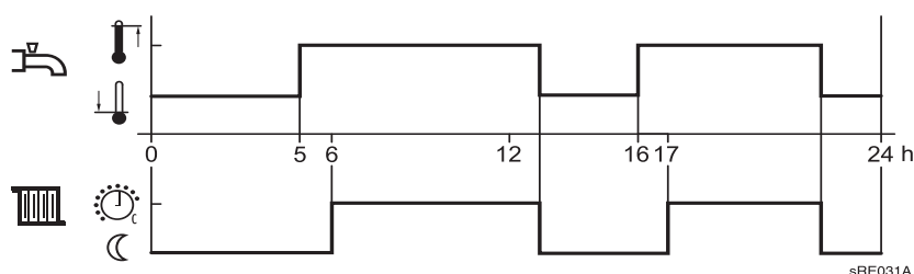
Rys. 17: Uruchamianie funkcji podgrzewania c.w.u. w zależności od programów sterowania zegarowego pracą obiegów c.o. (przykład)
