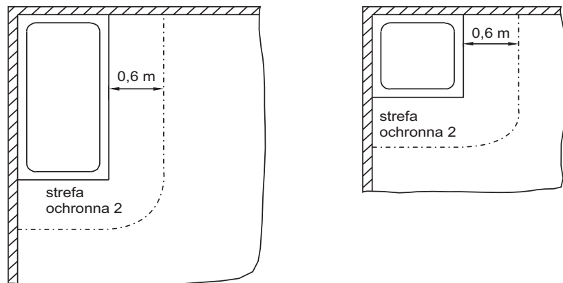
Rys. 3: Odległości od kotła BBK w łazienkach i pomieszczeniach z natryskami
