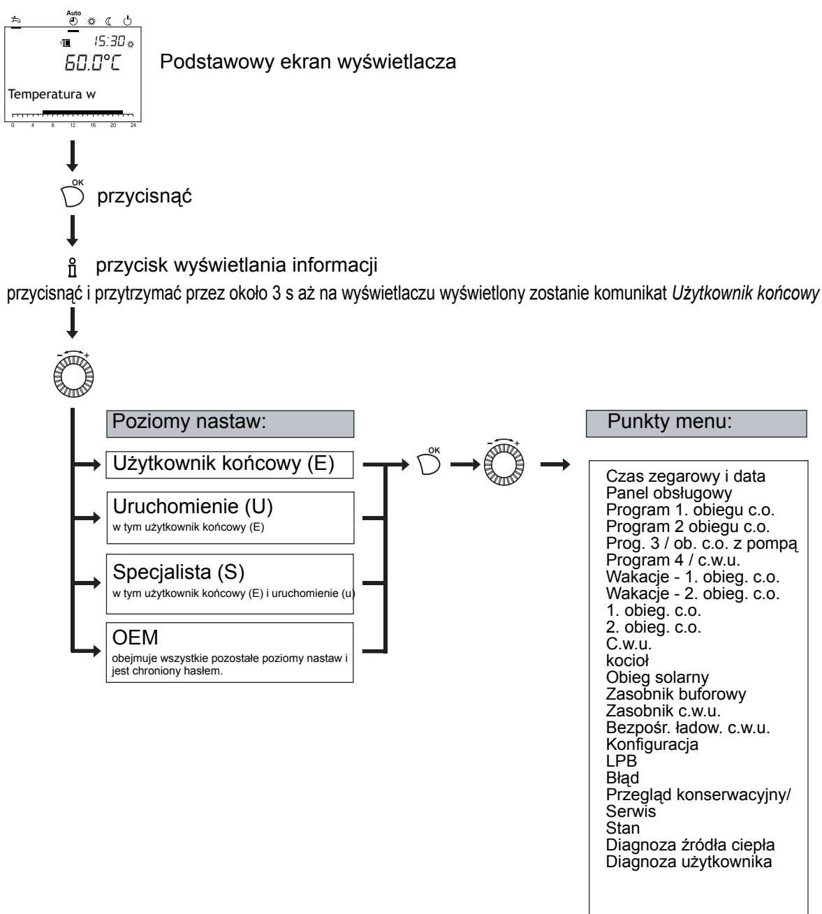
Rys. 13: Wybór poziomów nastaw i punktów menu
