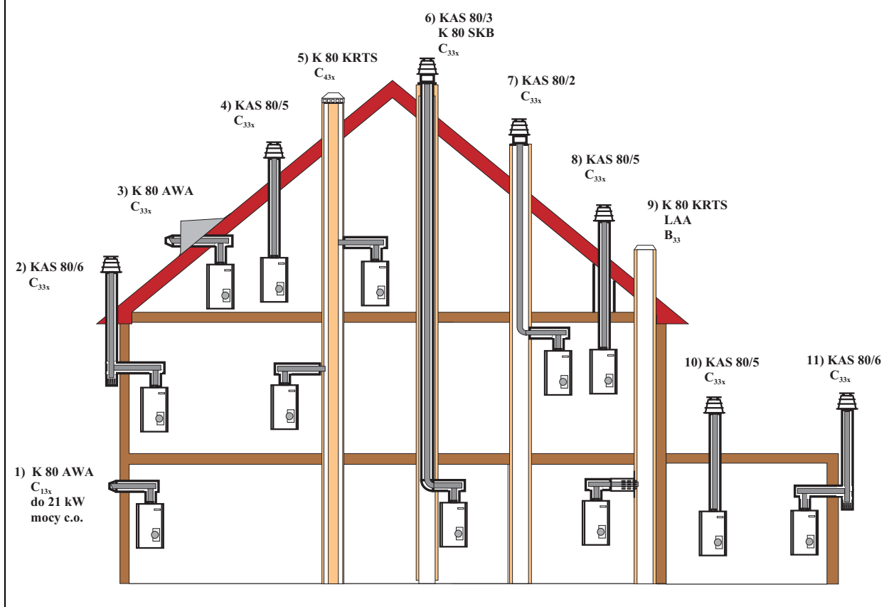
Rys. 5: Możliwości zamontowania kotła z zastosowaniem systemu KAS 80 (wyposażenie dodatkowe)
