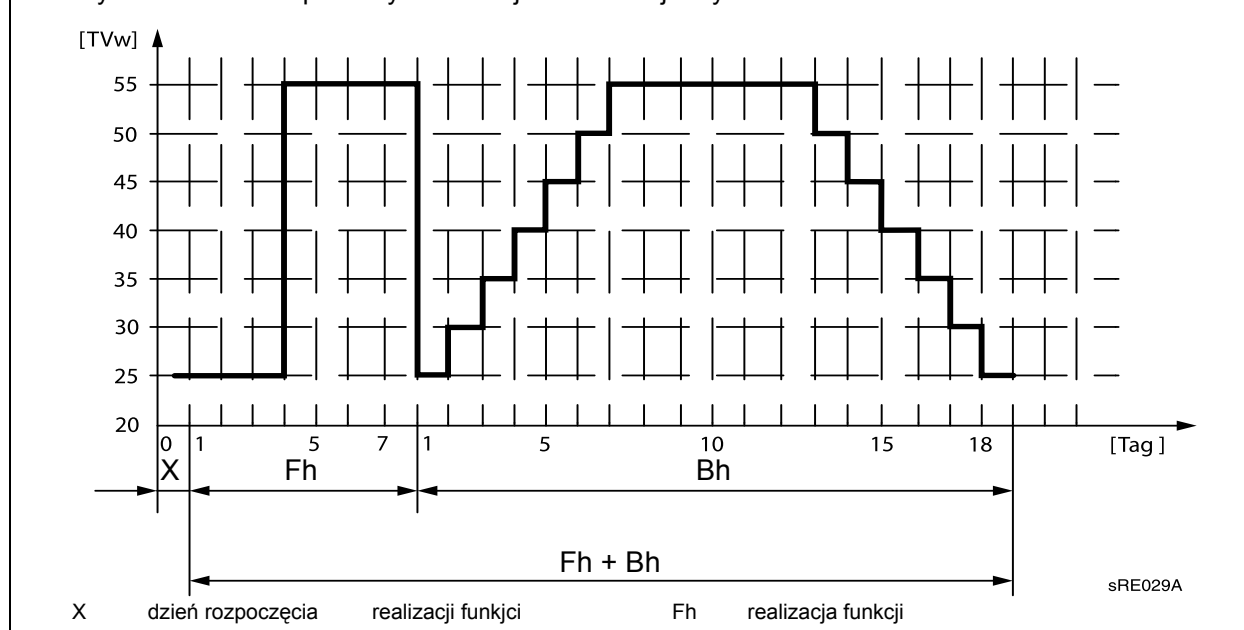
Rys. 15: Profil temperatury dla funkcji osuszania jastrychu
