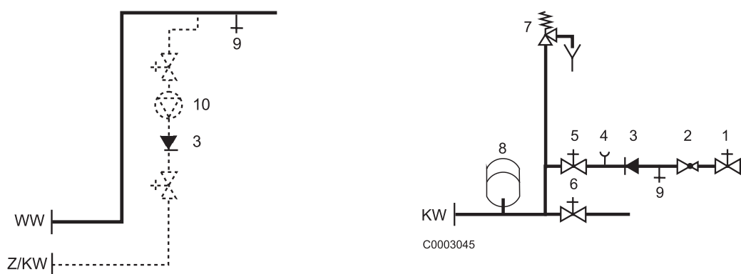
Rys. 9: Przyłącze zimnej wody zgodnie z normą DIN 1988
