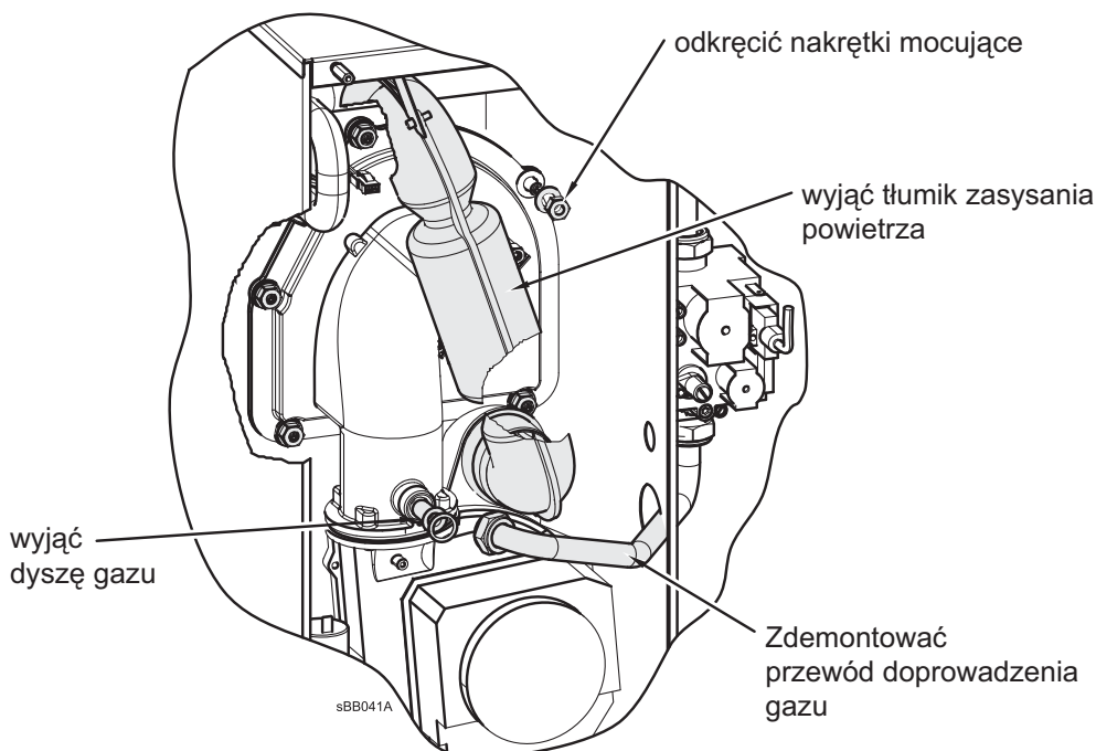
Rys. 30: Wymontowywanie palnika gazowego
