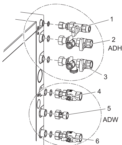
Rys. 8: Montaż zaworów odcinających
