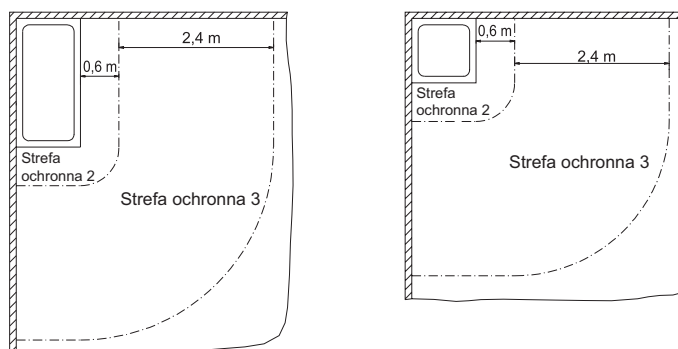
Rys. 3: Odległości w łazienkach i pomieszczeniach z natryskami
