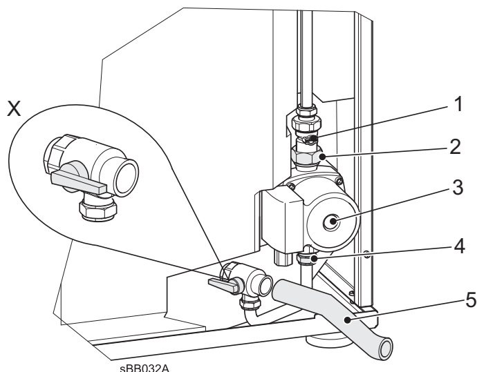
Rys. 34: Wymontowywanie pompy ładującej c.w.u.
