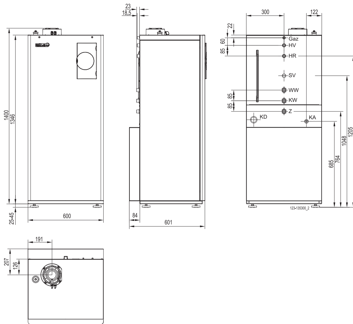
Rys. 1: Wymiary i przyłącza kotła
