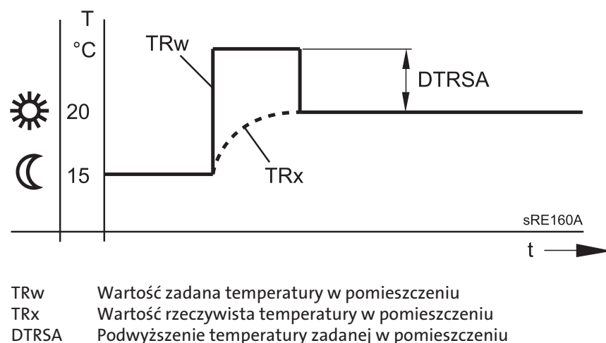
Rys. 20: Szybkie nagrzewanie
