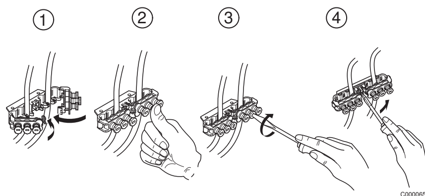
Rys. 14: Dławik kablowy
