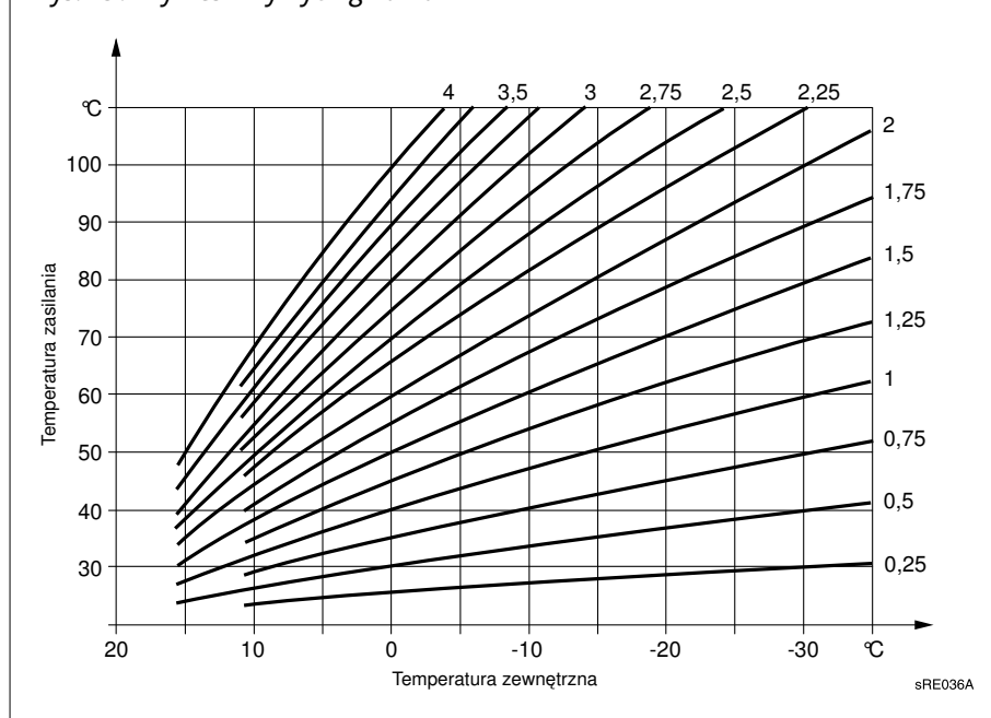
Rys. 19: Wykres krzywych grzania
