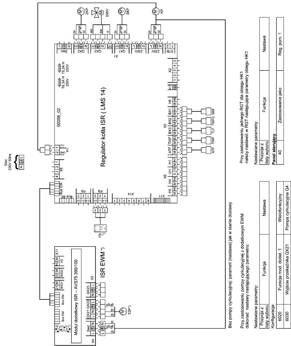
Rys. 5: Schemat połączeń elektrycznych
