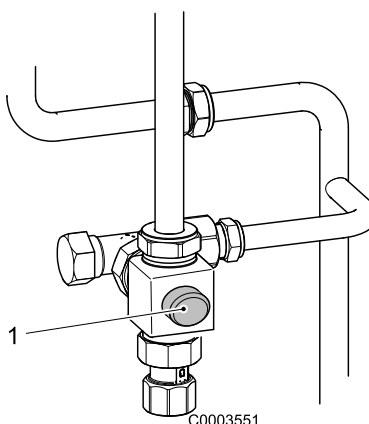
Rys. 10: Wstępna nastawa na zaworze mieszającym c.w.u.
