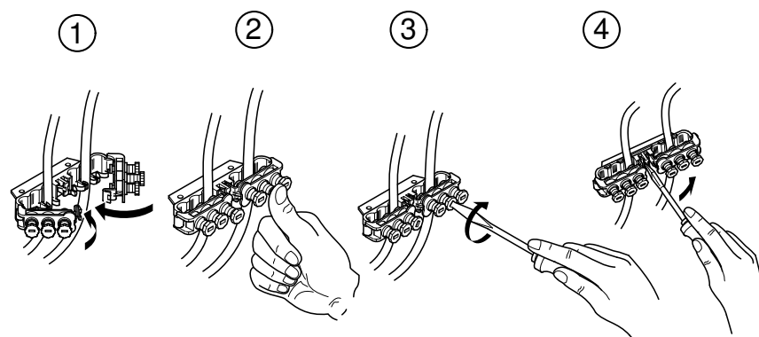
Rys. 16: Dławik kablowy
