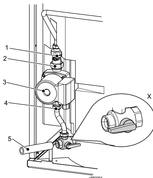
Rys. 39: Wymontowywanie pompy ładującej c.w.u.
