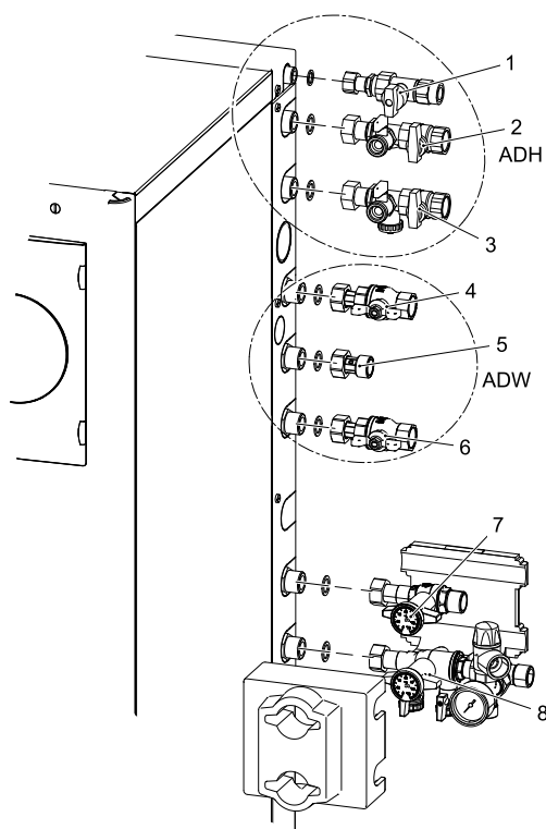
Rys. 8: Montaż zaworów odcinających
