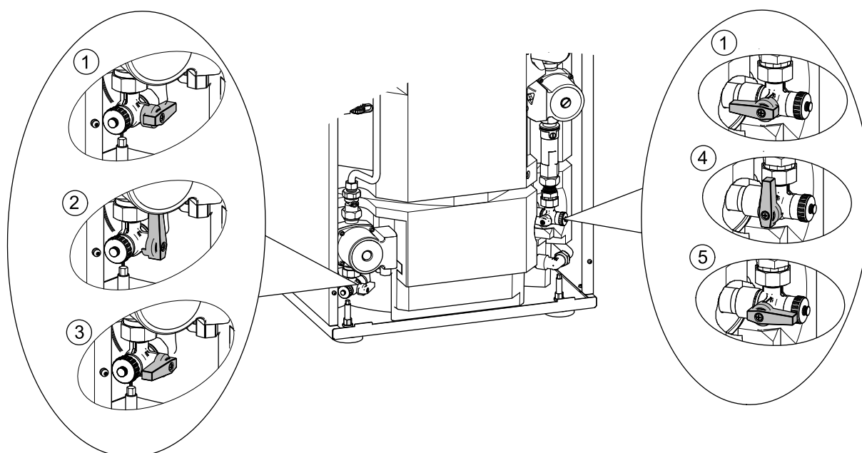
Rys. 38: Objasnienia do zaworów spustowych
