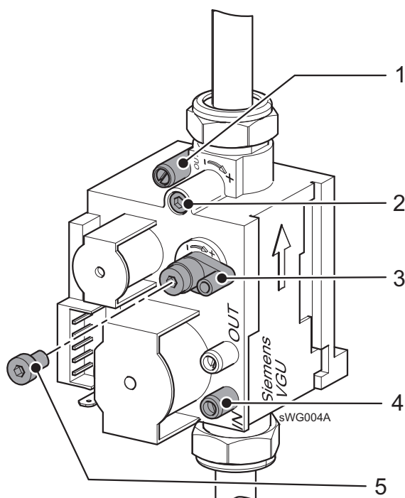
Rys. 10: Armatura gazowa (nastawa ciśnienia dyszy za pomocą klucza Torx T15)
