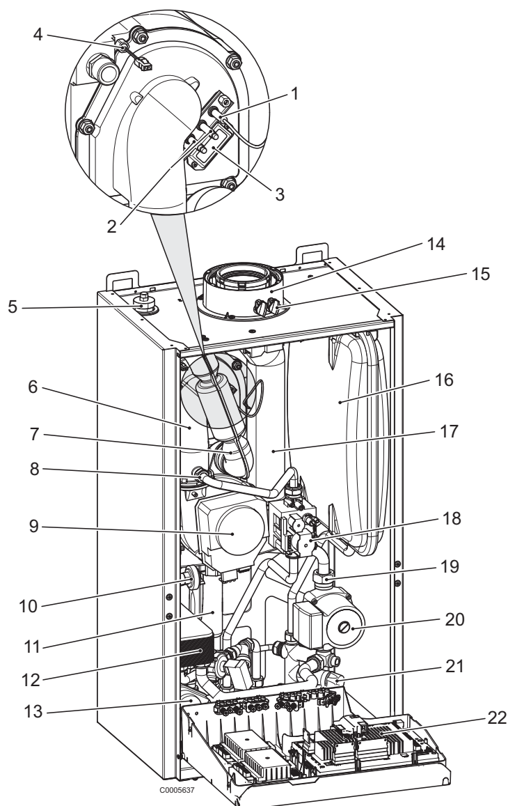
Rys. 27: Widok kotła WBC (na rysunku bez przedniej ścianki i pokrywy modułu regulacyjnego)
