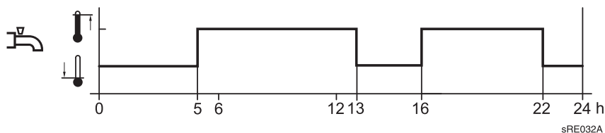
Rys. 23: Uruchamianie funkcji podgrzewania c.w.u. zgodnie z 4. programem sterowania zegarowego (przykład)
