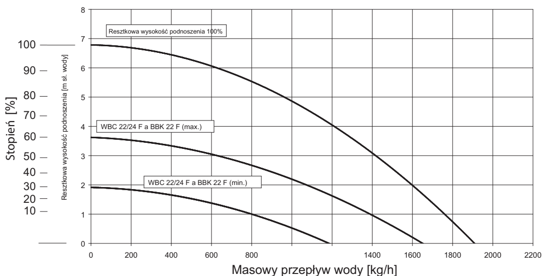
Rys. 21: Resztkowa wysokość podnoszenia WBC 22/24 E
