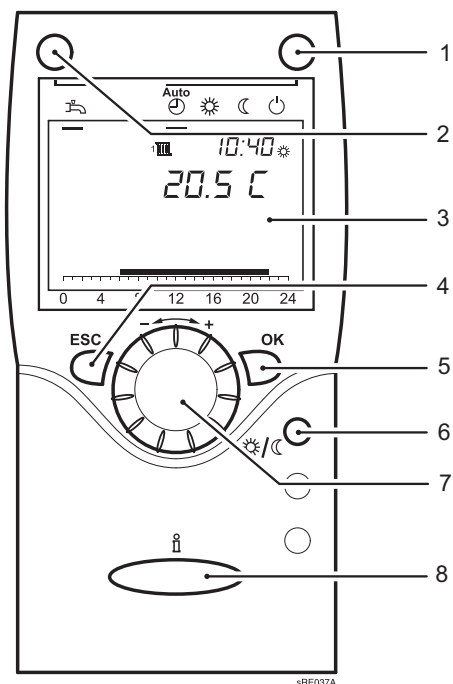
Rys. 25: Panel obsługi regulatorów RGT
