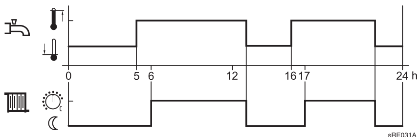
Rys. 22: Uruchamianie funkcji podgrzewania c.w.u. w zależności od programów sterowania zegarowego pracą obiegów c.o.(przykład)
