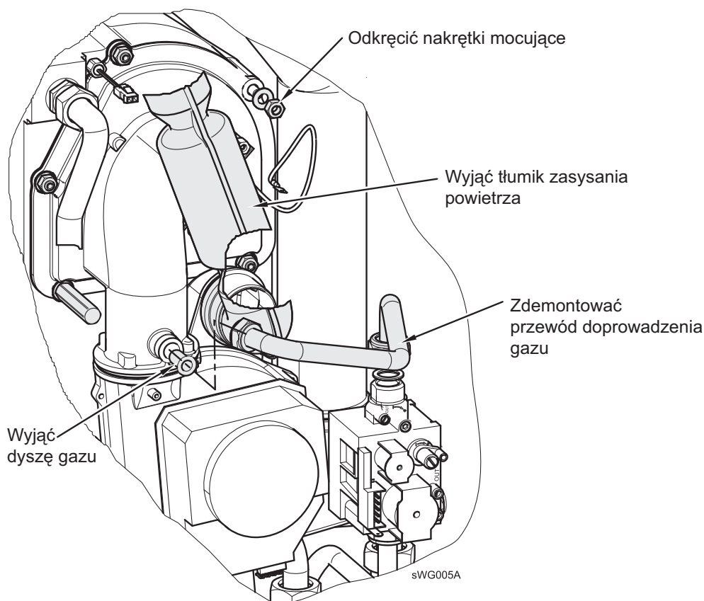
Rys. 26: Wymontowywanie palnika gazowego
