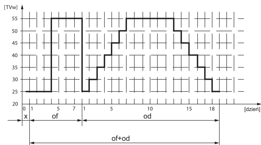
Rys. 20: Profil temperatury dla funkcji osuszania jastrychu
