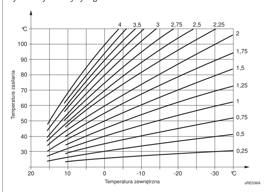
Rys. 14: Wykres krzywych grzania
