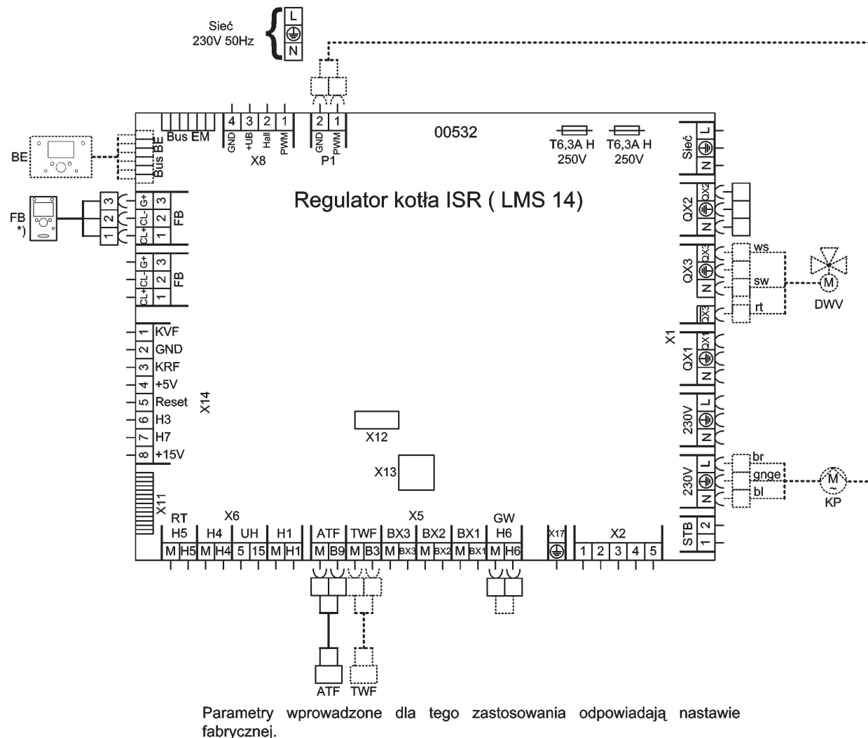
Rys. 5: Schemat połączeń elektrycznych
