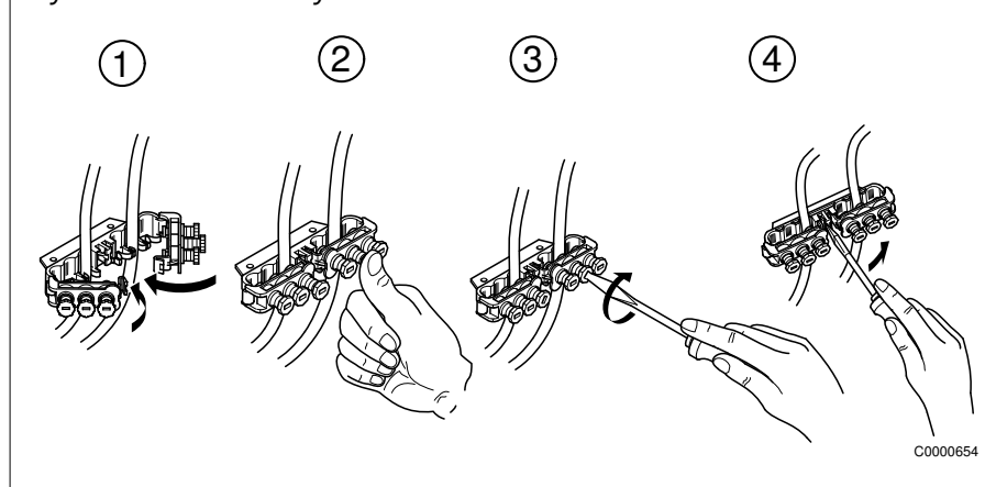
Rys. 15: Dławik kablowy
