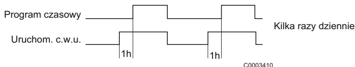
Rys. 29: Wyprzedzenie ładowania
