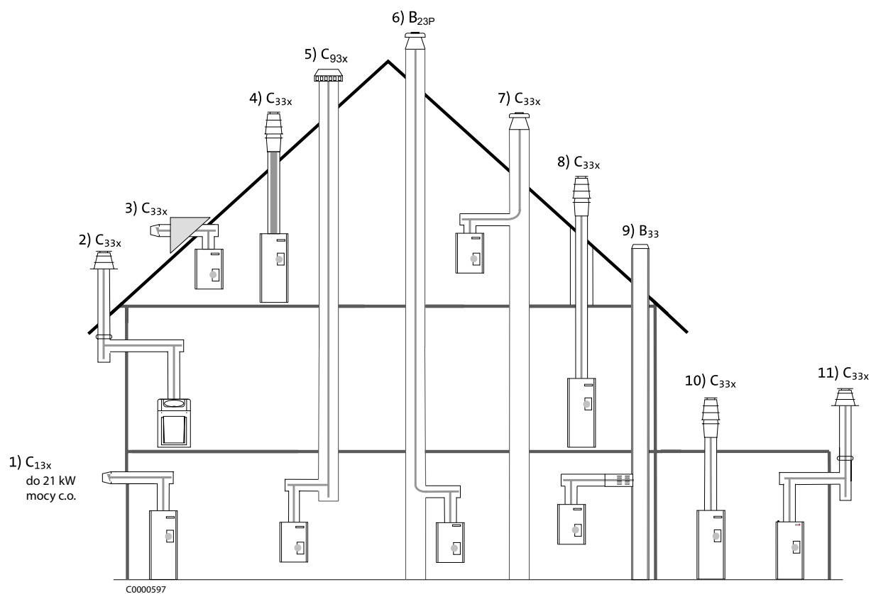
Rys. 10: Możliwości zamontowania kotła z zastosowaniem systemu KAS (wyposażenie dodatkowe)
