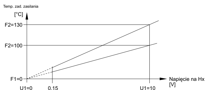
Rys. 30: Przykład zapotrzebowania na ciepło 10 V i na chłód 10 V
