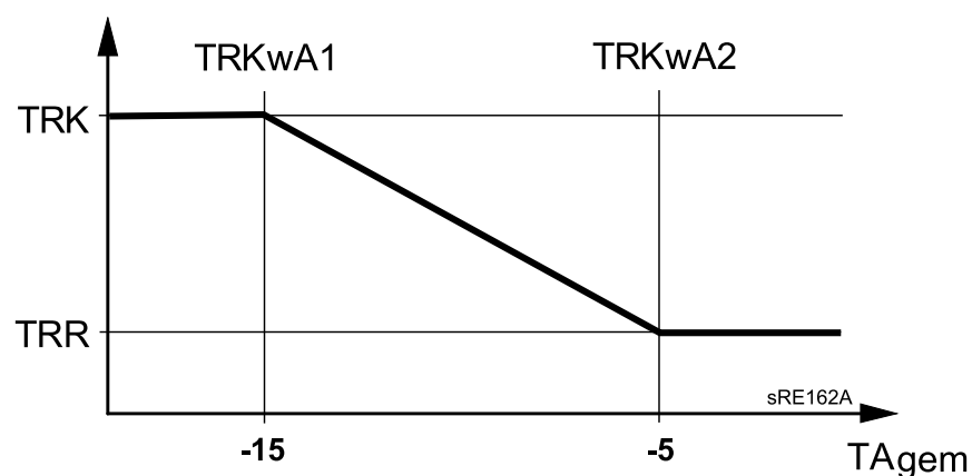
Rys. 23: Zred. obniż.
