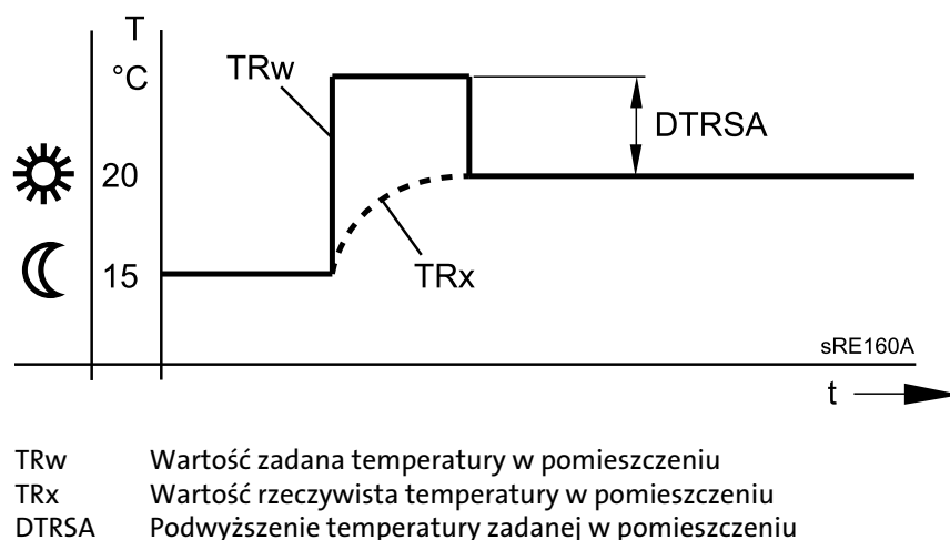
Rys. 21: Szybkie nagrzewania
