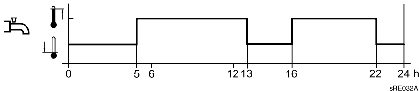
Rys. 27: Uruchamianie funkcji podgrzewania c.w.u. zgodnie z 4. programem sterowania zegarowego (przykład)
