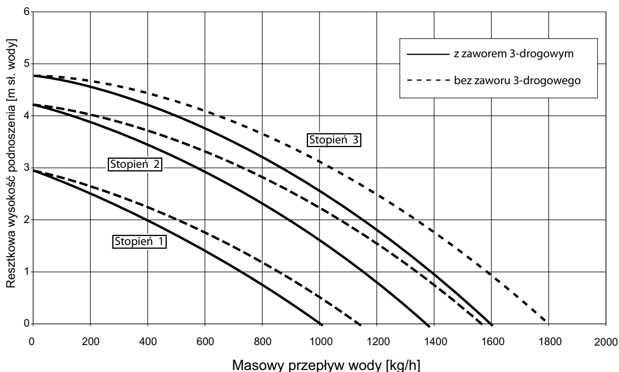
Rys. 25: Resztkowa wysokość podnoszenia WBK 20 E
