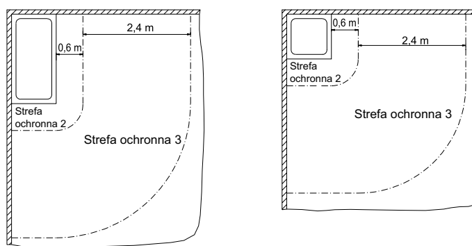
Rys. 4: Odległości w łazienkach i pomieszczeniach z natryskami
