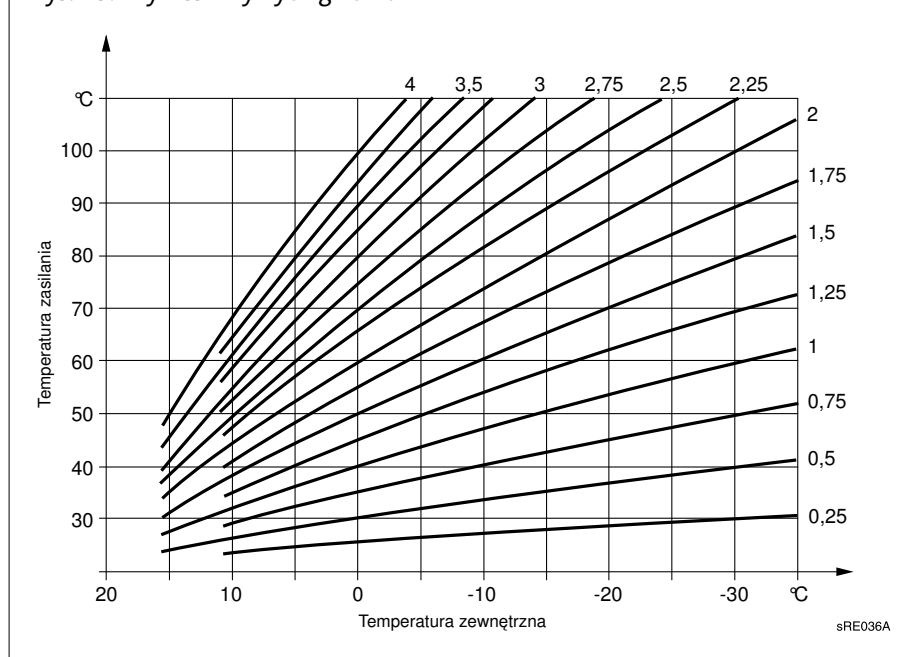
Rys. 18: Wykres krzywych grzania
