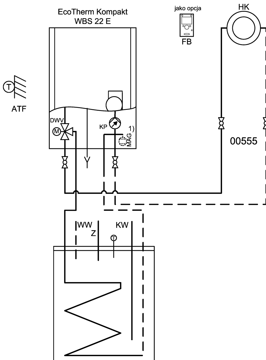
Rys. 4: Przykład: obieg c.o. z pompą obiegową, z regulatorem pokojowym oraz układem regulacji temperatury w podgrzewaczu c.w.u.
