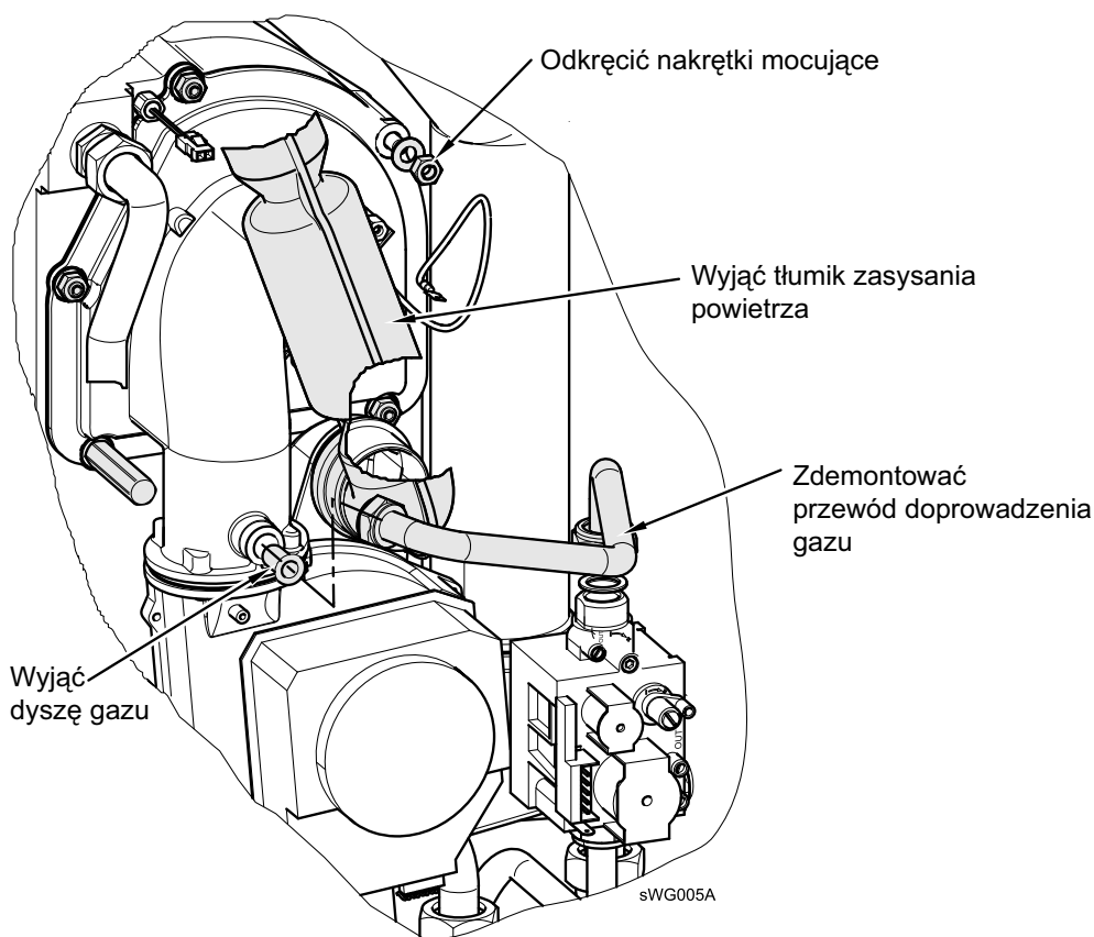
Rys. 29: Wymontowywanie palnika gazowego
