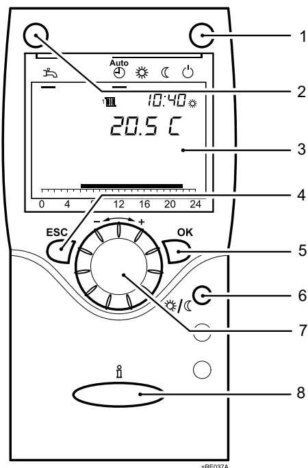
Rys. 28: Panel obsługi regulatorów RGT
