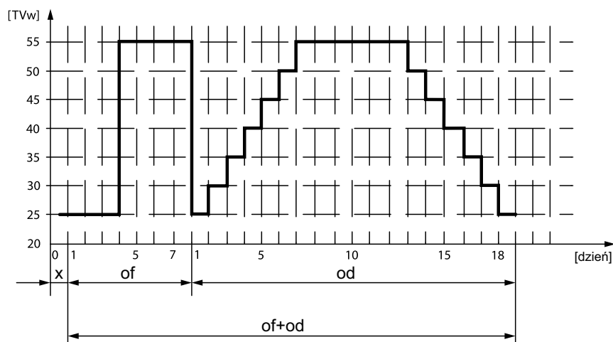
Rys. 22: Profil temperatury dla funkcji osuszania jastrychu
