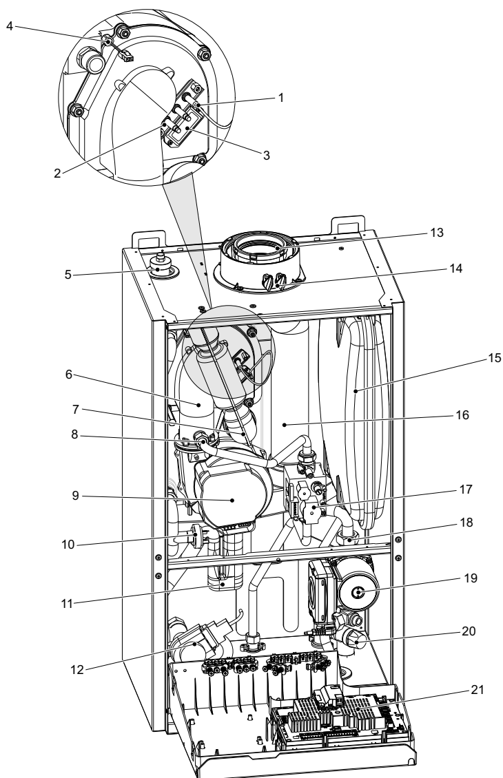
Rys. 30: Widok kotła WBS (na rysunku bez przedniej ścianki obudowy i pokrywy modułu regulacyjnego)
