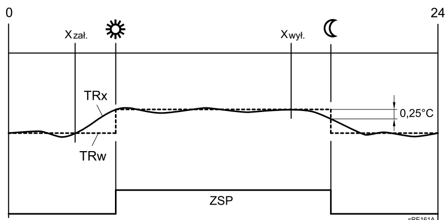
Rys. 20: Optymalizacja załączania i wyłączenia
