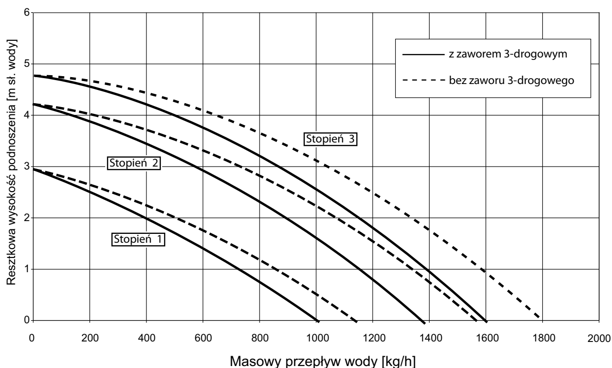
Rys. 23: Resztkowa wysokość podnoszenia WBS 14/22 E
