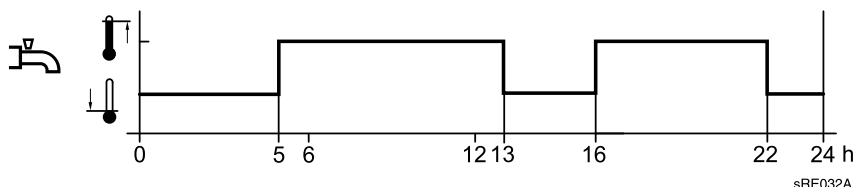
Rys. 25: Uruchamianie funkcji podgrzewania c.w.u. zgodnie z 4. programem sterowania zegarowego (przykład)
