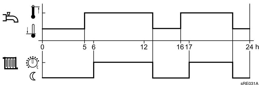
Rys. 24: Uruchamianie funkcji podgrzewania c.w.u. w zależności od programów sterowania zegarowego pracą obiegów c.o.(przykład)
