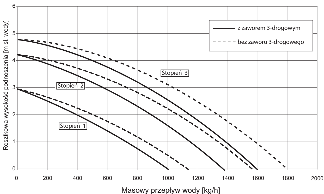
Rys. 24: Resztkowa wysokość podnoszenia WBS 14 - 22 E
