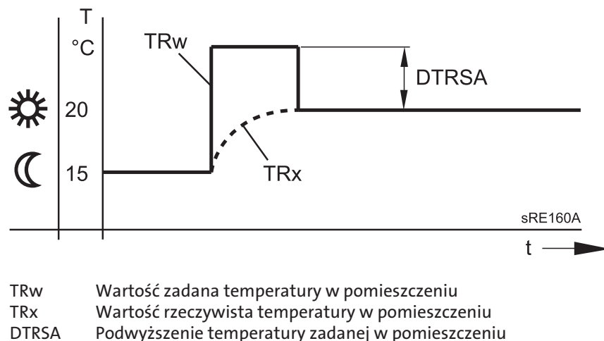
Rys. 20: Szybkie nagrzewanie
