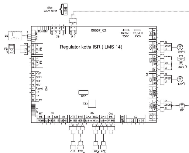
Rys. 9: Schemat połączeń elektrycznych
