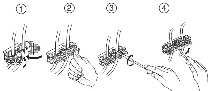
Rys. 14: Dławik kablowy
