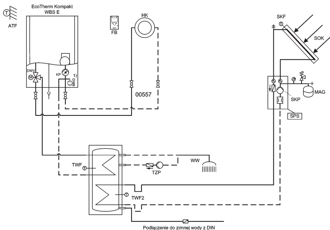
Rys. 8: Przykład: jeden obieg c.o. z pompą obiegową, z regulatorem pokojowym i solarnym podgrzewaczem c.w.u.
