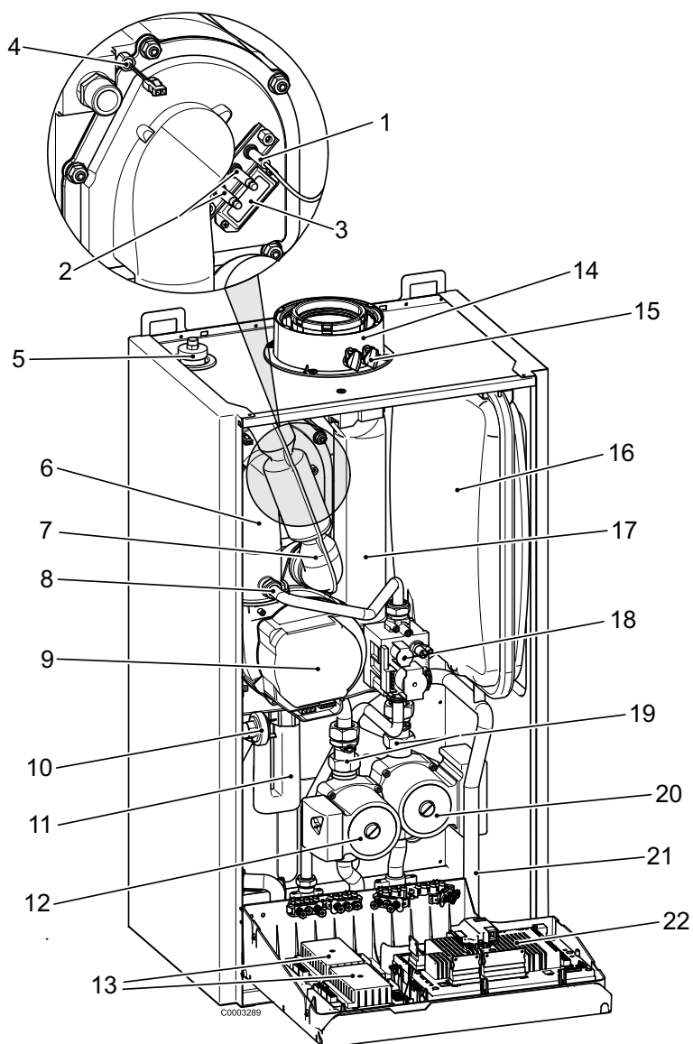
Rys. 35: Widok kotła WGB (na rysunku bez przedniej ścianki i pokrywy modułu regulacyjnego)
