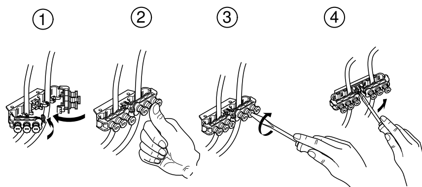
Rys. 14: Dławik kablowy
