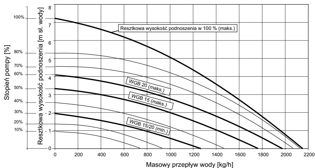
Rys. 24: Resztkowa wysokość podnoszenia w kotle WGB 15-38 E
