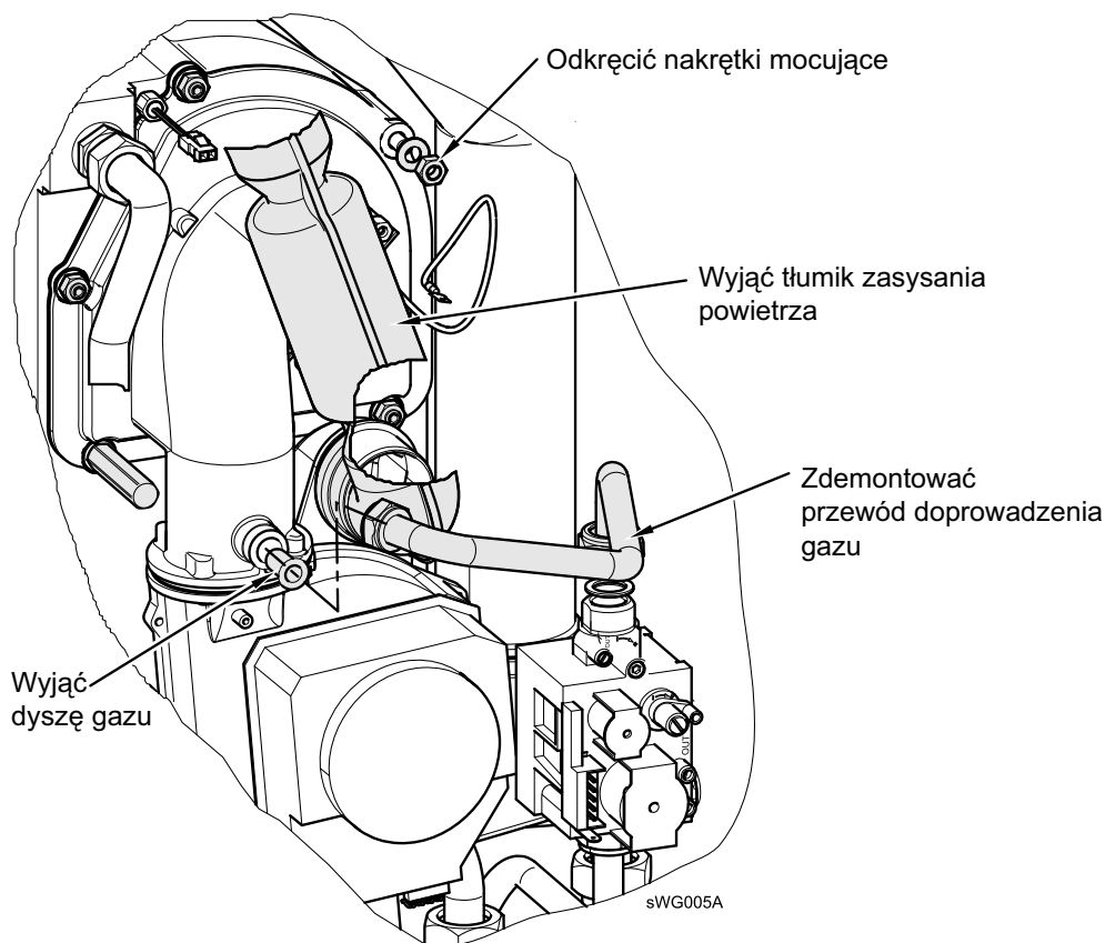
Rys. 34: Wymontowywanie palnika gazowego
