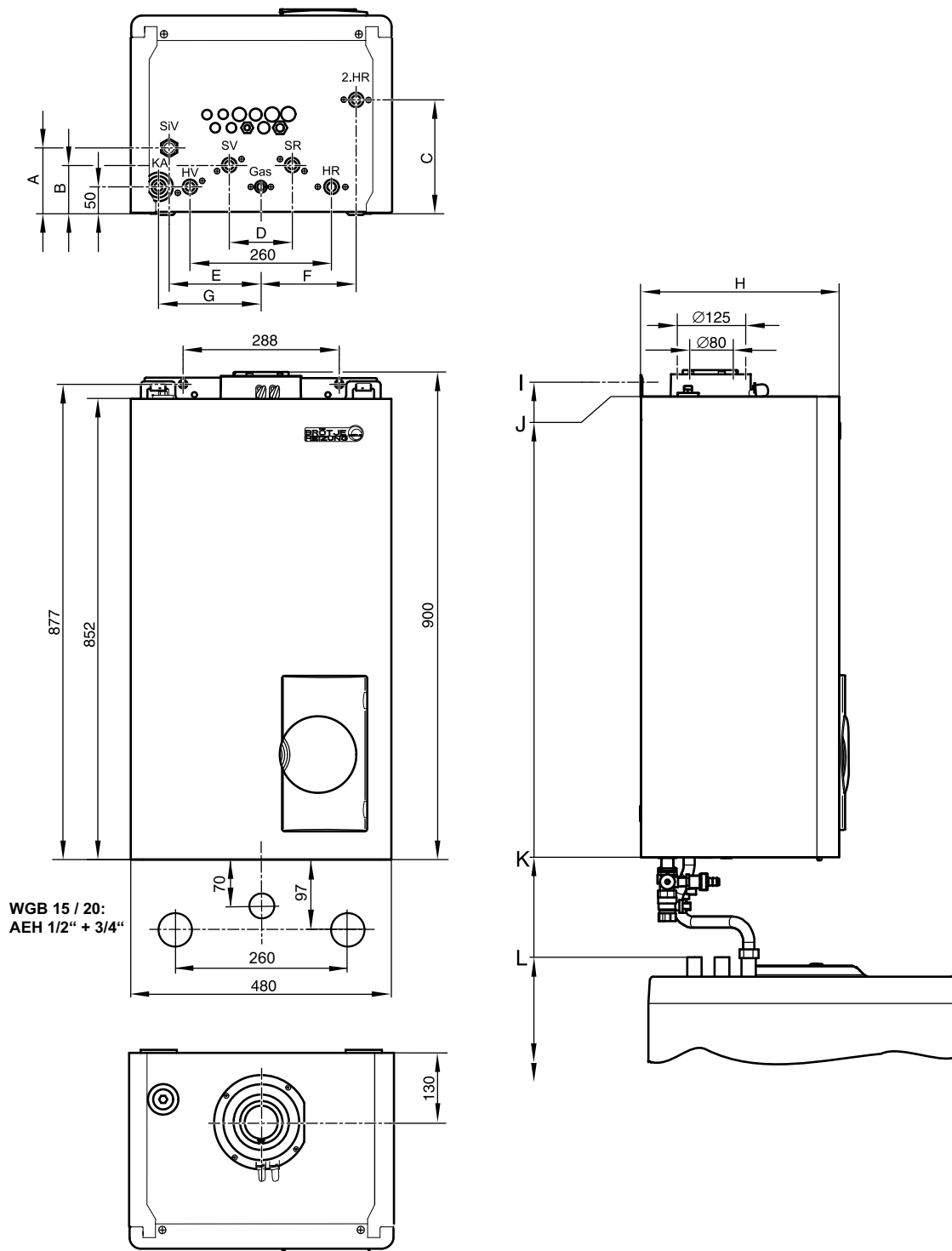
Rys. 1: Wymiary i przyłącza
