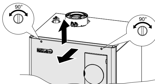
Rys. 6: Zdejmowanie przedniej obudowy kotła
