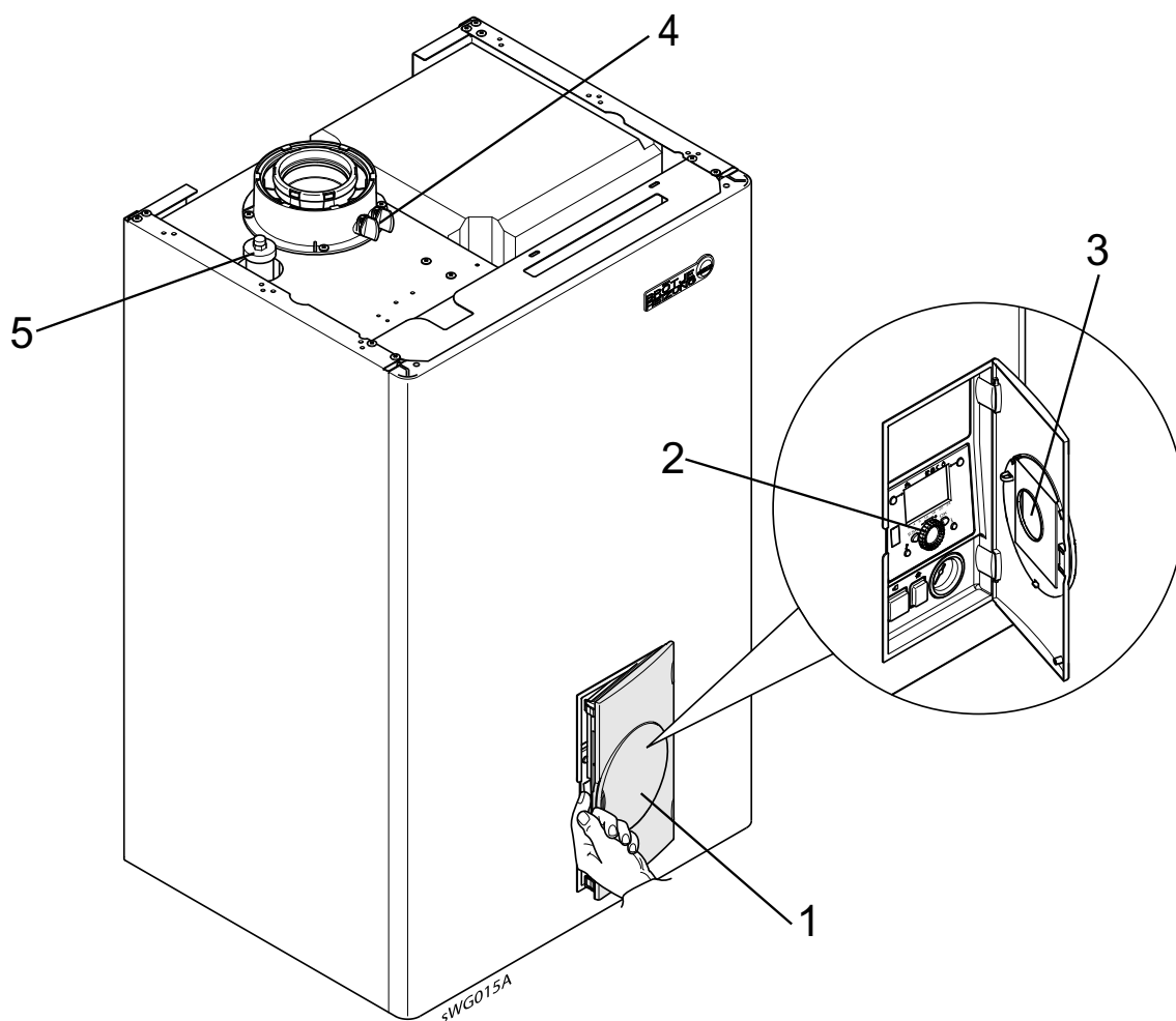
Rys. 1: Rysunek poglądowy kotła WBK
