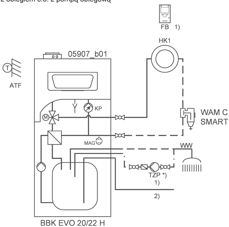
Rys.9 kocioł BBK EVO z obiegiem c.o. z pompą obiegową
