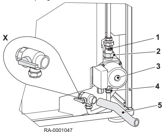
Rys.43 Wymontowywanie pompy ładującej podgrzewacz c.w.u.
