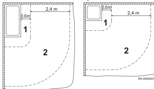
Rys.8 Odległości w łazienkach i pomieszczeniach z natryskami
