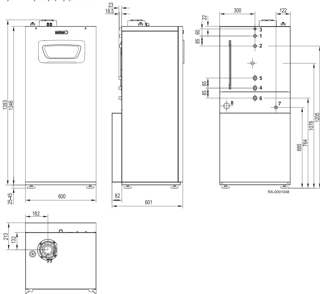
Rys.2 Wymiary i przyłącza kotła BBK EVO
