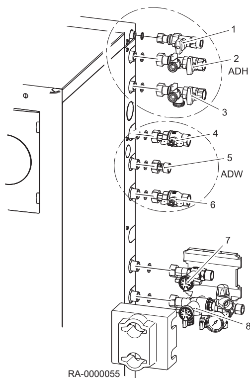
Rys.13 Montaż zaworów odcinających
