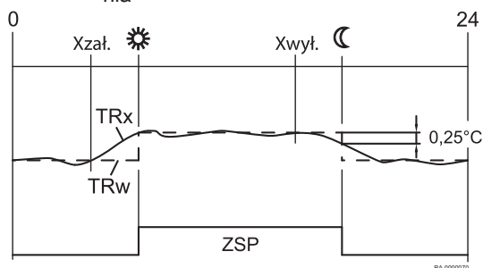
Rys.30 Optimalizacja załączania i wyłączania
