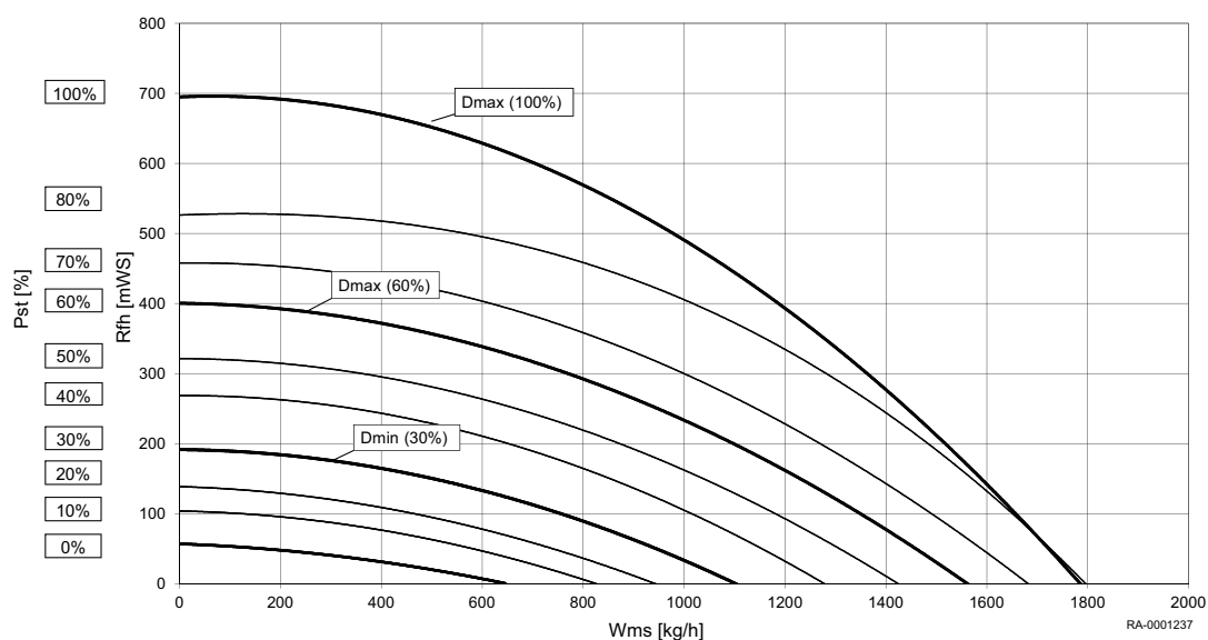
Rys.1 Łączne ciśnienie dynamiczne BBK EVO 20/22
