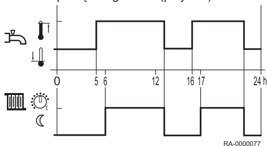
Rys.33 Uruchamianie w zależności od programów sterowania zegarowego pracą obiegów c.o. (przykład)
