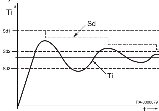
Rys.35 Histereza
