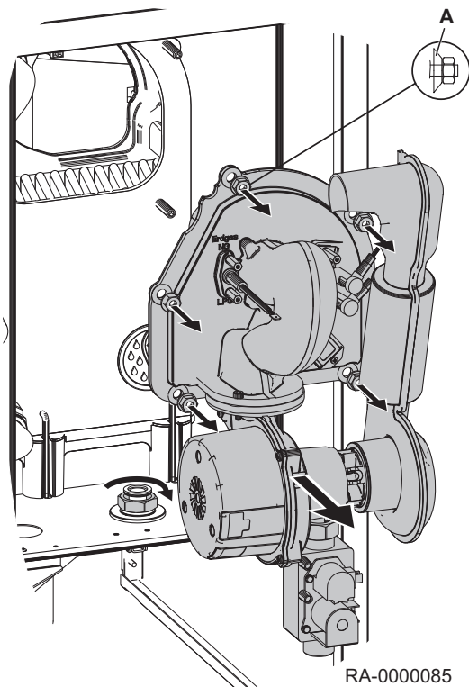
Rys.41 Wymontowywanie palnika gazowego
