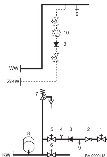
Rys.14 Podłączenie zimnej wody zgodnie z DIN 1988
