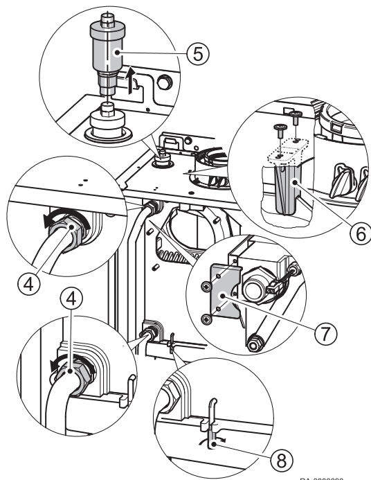
Rys.42 Wymontowywanie wymiennika ciepła
