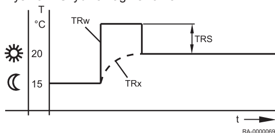
Rys.19 Szybkie nagrzewanie
