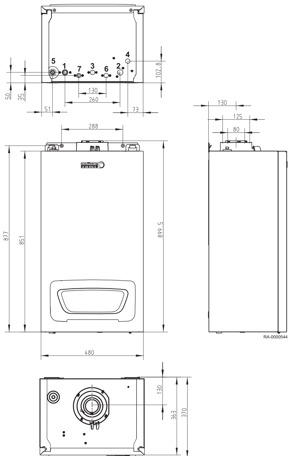
Rys.1 Wymiary i przyłącza kotła WBC
