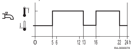
Rys.22 Uruchamianie zgodnie z 4. programem sterowania zegarowego (przykład)
