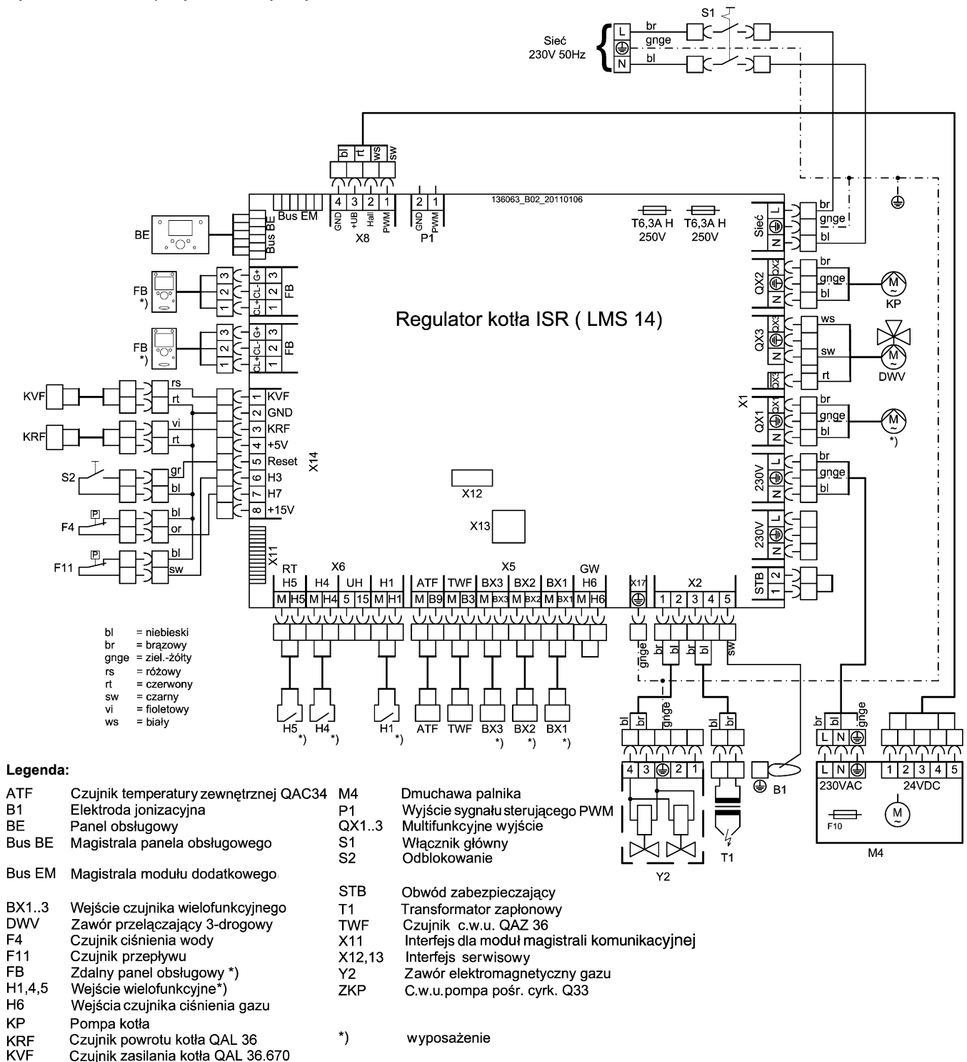
Rys.2 Schemat połączeń elektrycznych WBC
