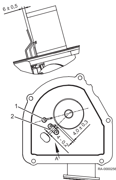
Rys.24 Elektrody
