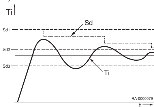
Rys.33 Histereza
