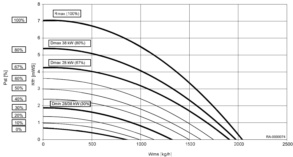
Rys.2 Łączne ciśnienie dynamiczne WGB EVO 28
