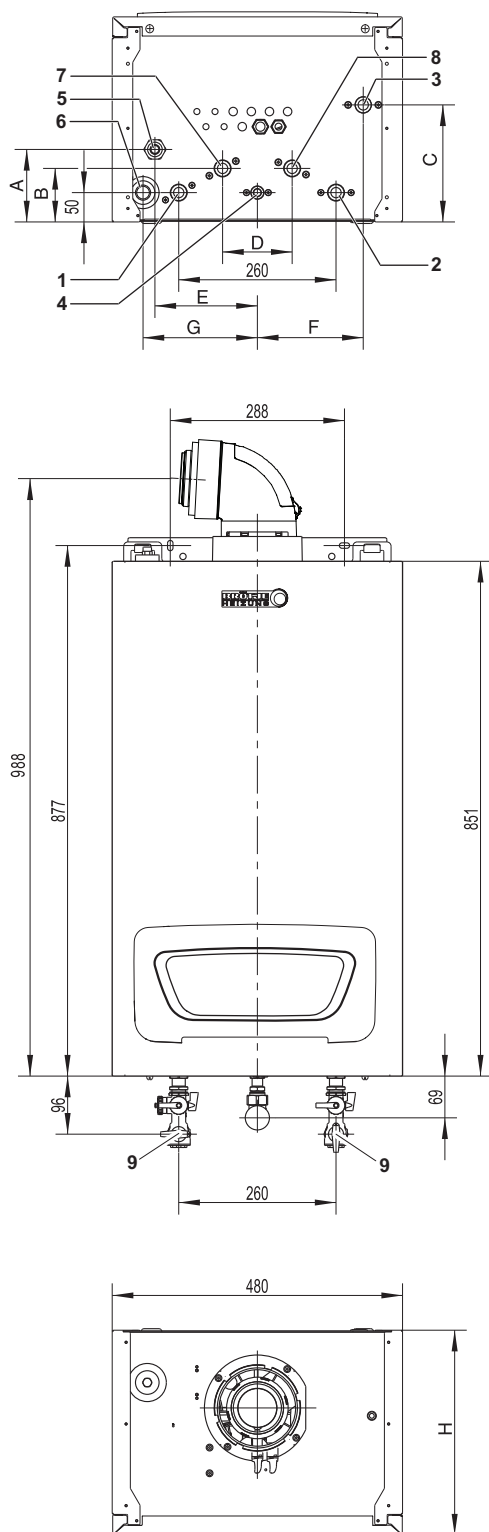
Rys.3 Wymiary i przyłącza kotła WGB EVO
