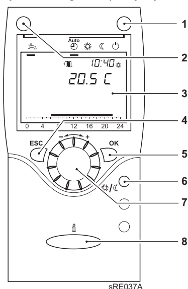
Rys.7 Regulator pokojowy RGT
