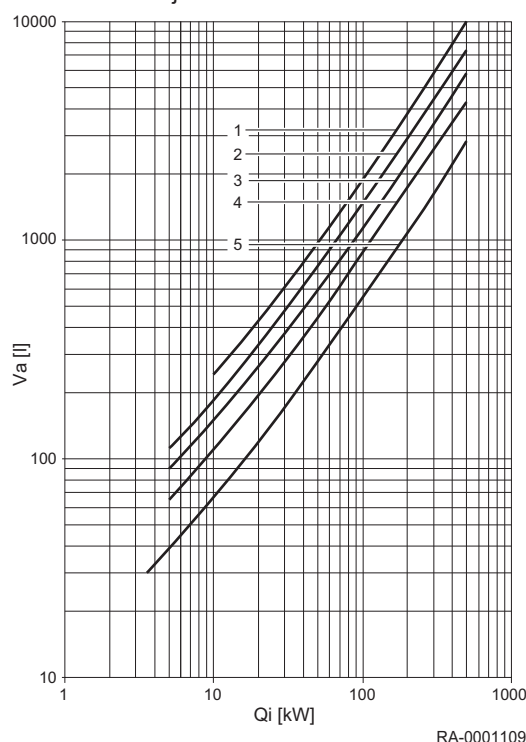
Rys.8 Określanie pojemności wodnej instalacji
