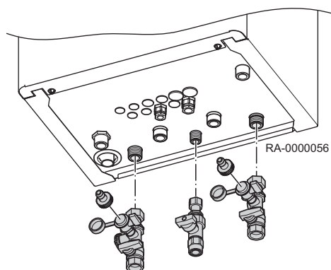
Rys.12 Montaż zaworów odcinających
