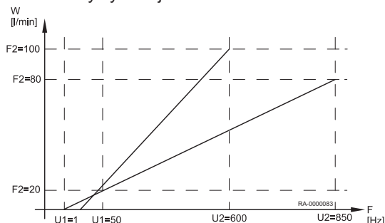
Rys.37 Przykład dwóch różnych charakterystyk czujnika
