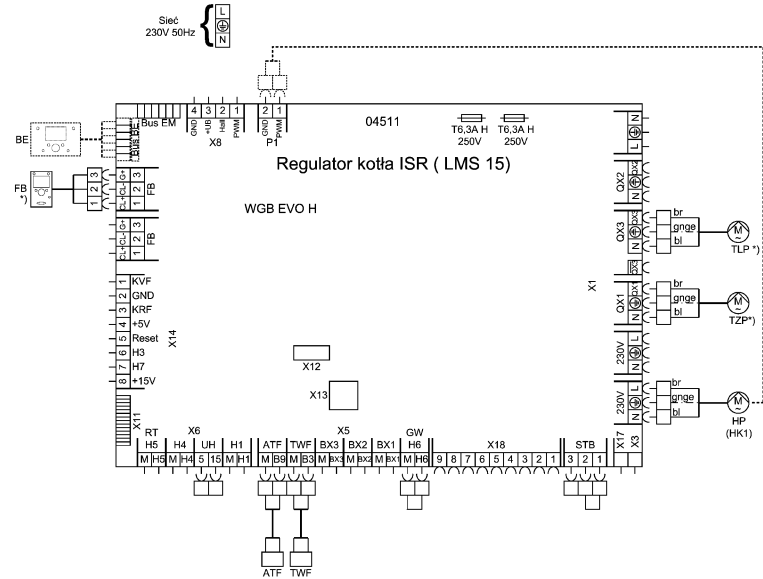
Rys.11 Schemat elektryczny
