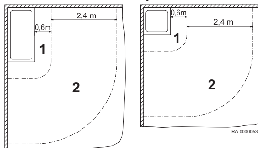
Rys.9 Odległości w łazienkach i pomieszczeniach z natryskami
