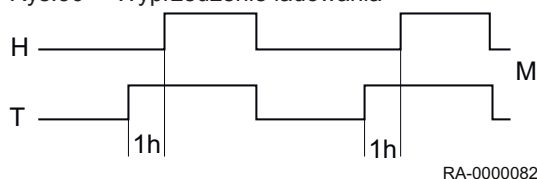
Rys.36 Wyprzedzenie ładowania
