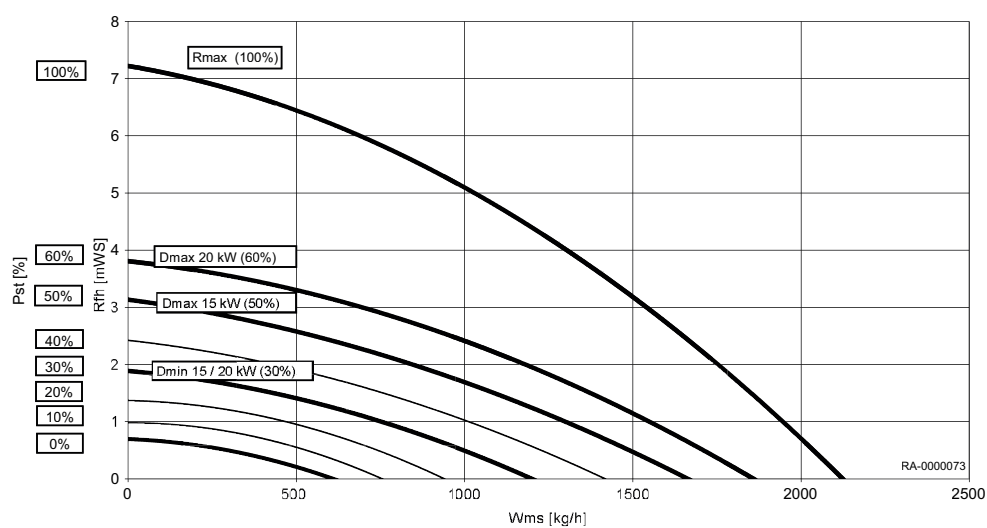
Rys.1 Łączne dynamiczne WGB EVO 15 — 20
