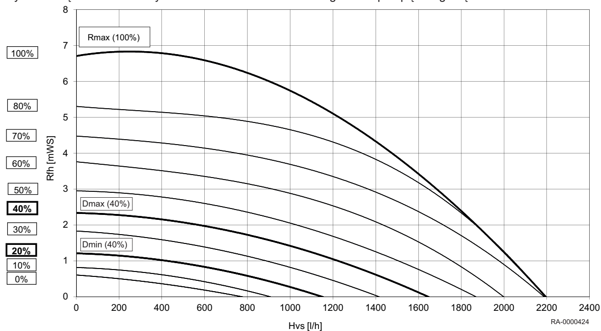
Rys.1 Łączne ciśnienie dynamiczne WGB-M EVO dla obiegu c.o. z pompą obiegową
