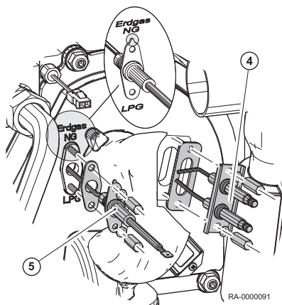
Rys.43 Wymontowywanie elektrody zapłonowej i jonizacyjnej
