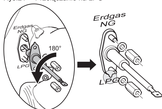
Rys.21 Przelączenie na LPG
