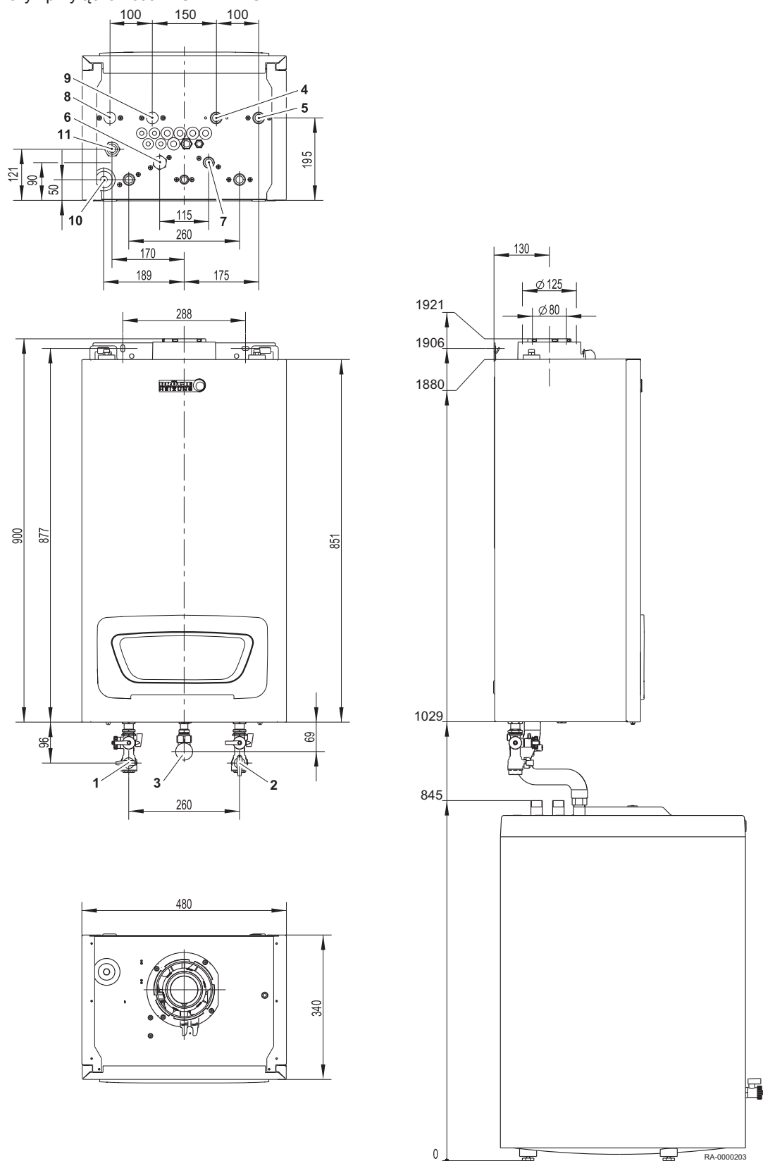
Rys.4 Wymiary i przyłącza kotła WGB-M EVO
