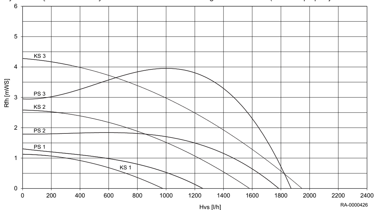
Rys.3 Łączne ciśnienie dynamiczne WGB-M EVO dla obiegu z mieszaczem (ciśnienie proporcjonalne lub stałe, stopień 1–3)
