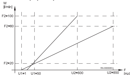
Rys.39 Przykład dwóch różnych charakterystyk czujnika
