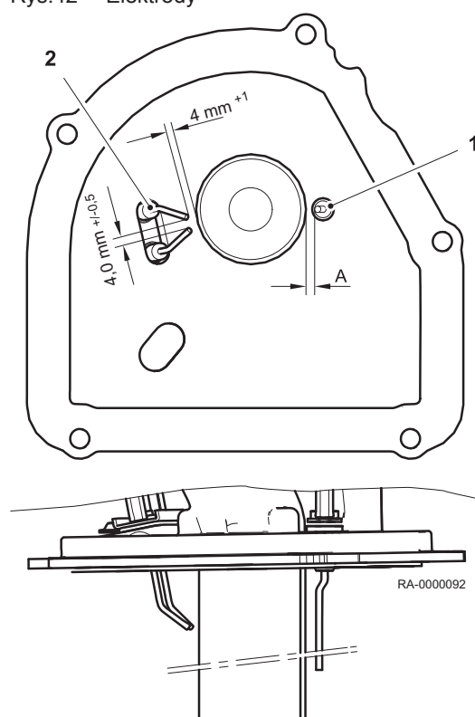
Rys.42 Elektrody
