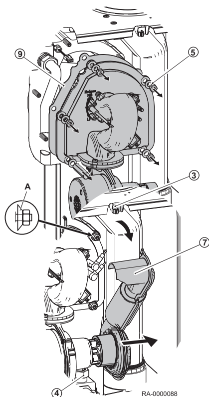
Rys.44 Wymontowywanie palnika gazowego
