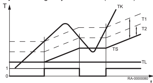
Rys.36 Regulacja ładowania (schemat)
