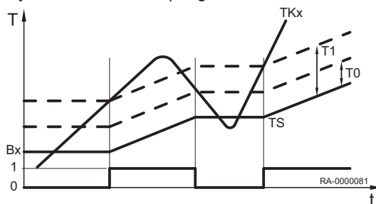
Rys.37 Ładowanie podgrzewacza
