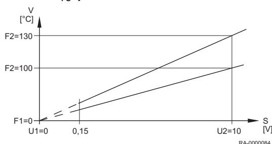
Rys.40 Przykład zapotrzebowania na ciepło 10 V
