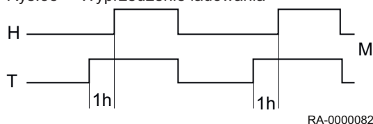
Rys.38 Wyprzedzenie ładowania
