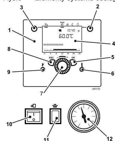
Rys.6 Elementy systemu obsługi
