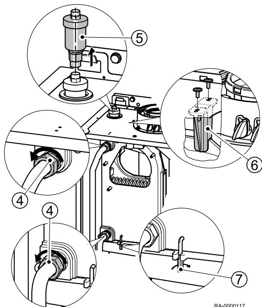
Rys.45 Wymontowywanie wymiennika ciepła
