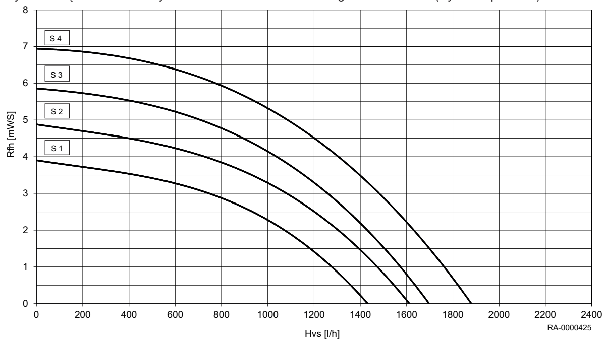
Rys.2 Łączne ciśnienie dynamiczne WGB-M EVO dla obiegu z mieszaczem (wybór stopnia 1–4)
