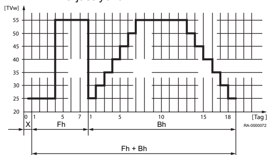
Rys.32 Profil temperaturowy funkcji suszenia jastrychu
