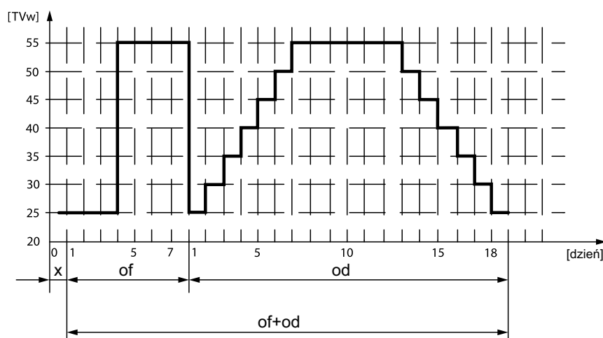
Rys. 23: Profil temperatury dla funkcji osuszania jastrychu
