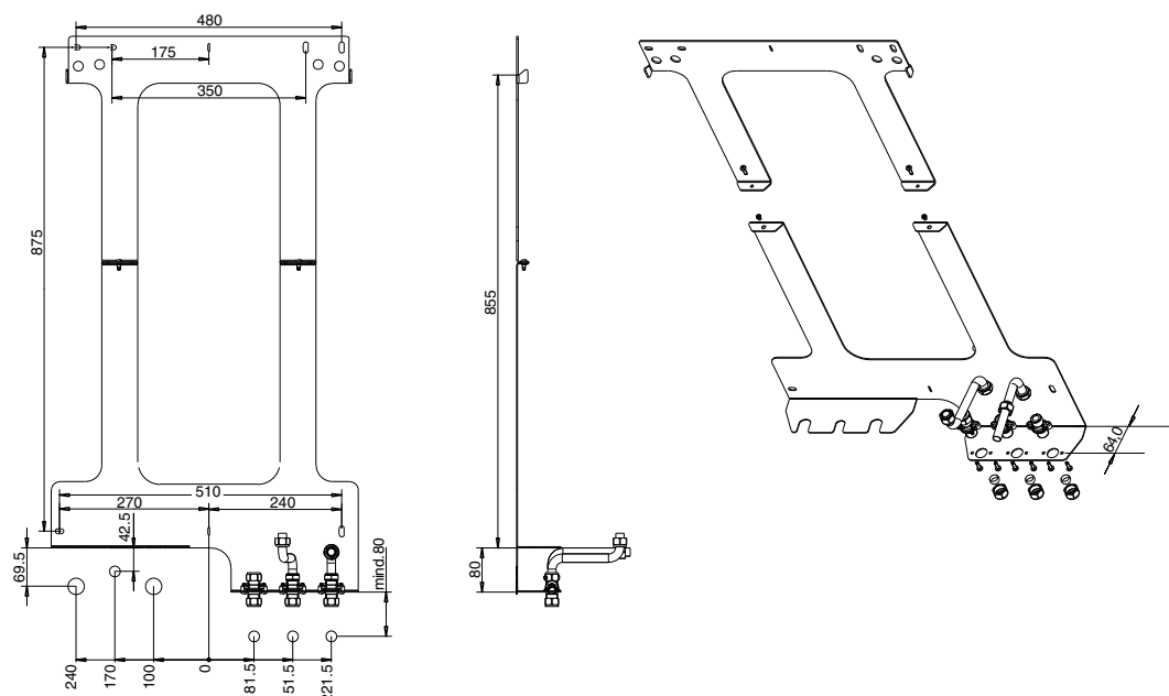
Rys. 2: Rama do szybkiego montażu SMR-KC *) kotła WGB-K
