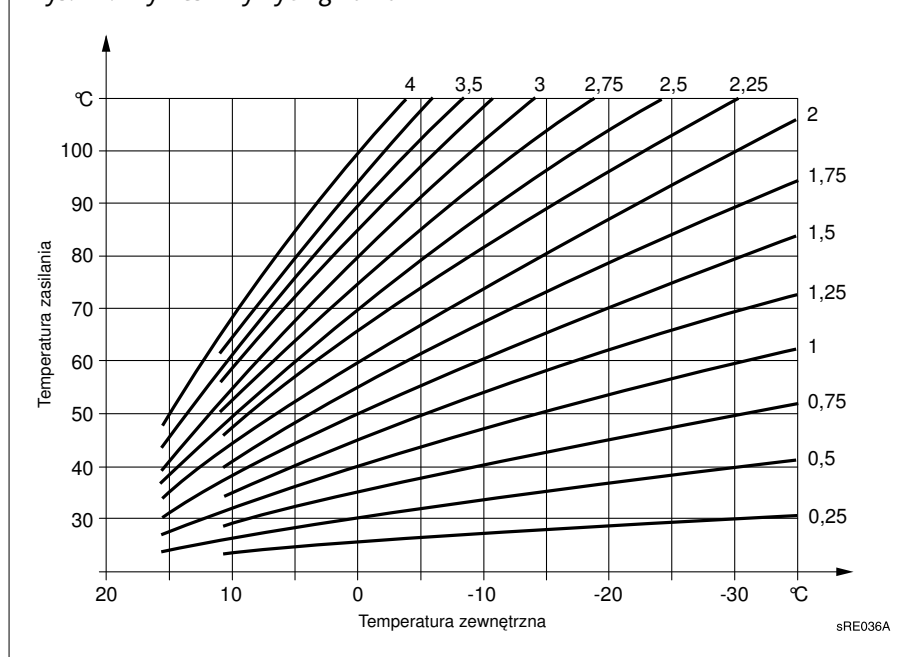
Rys. 17: Wykres krzywych grzania
