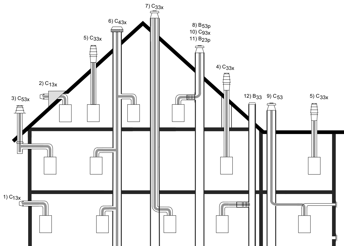
Rys. 10: Możliwości zamontowania kotła z zastosowaniem systemu KAS (wyposażenie dodatkowe)
