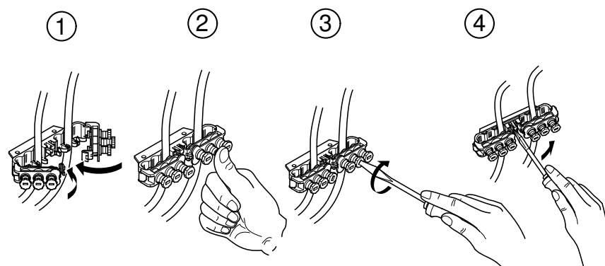
Rys. 14: Dławik kablowy
