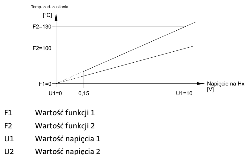
Rys. 29: Przykład zapotrzebowania na ciepło 10 V i na chłód 10 V
