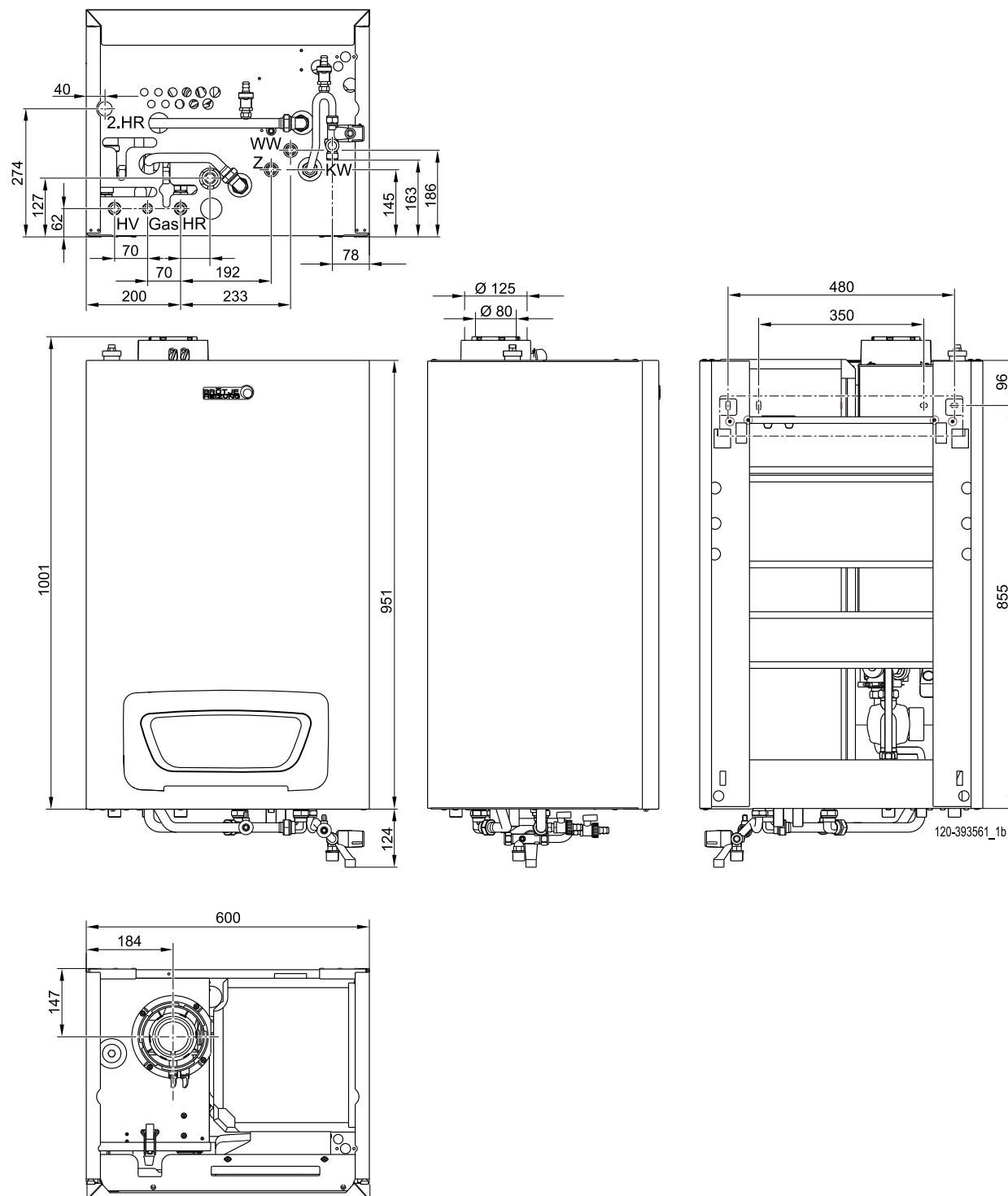
Rys. 1: Wymiary i przyłącza kotła EcoTherm Plus WGB-K
