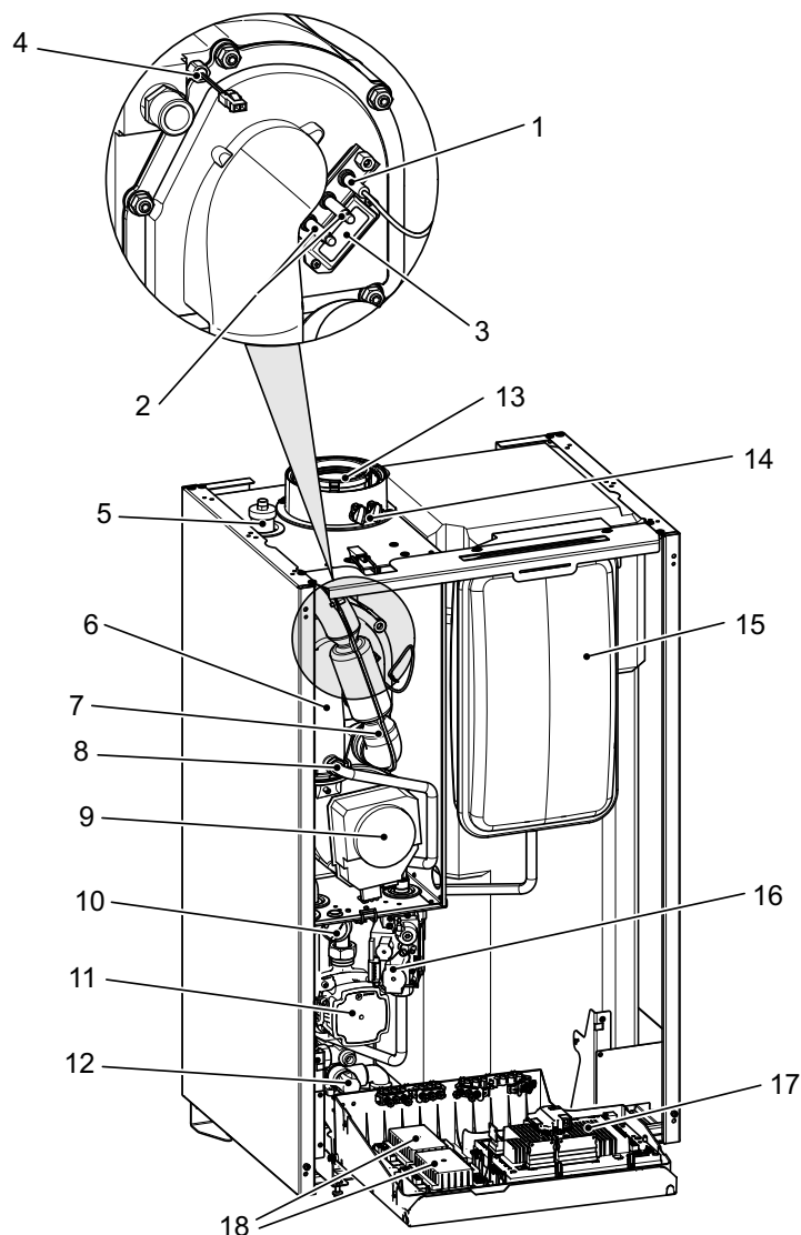
Rys. 32: Widok kotła WGB-K (na rys. bez przedniej ścianki i osłony modułu regulacyjnego)
