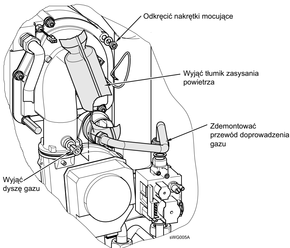
Rys. 31: Wymontowywanie palnika gazowego
