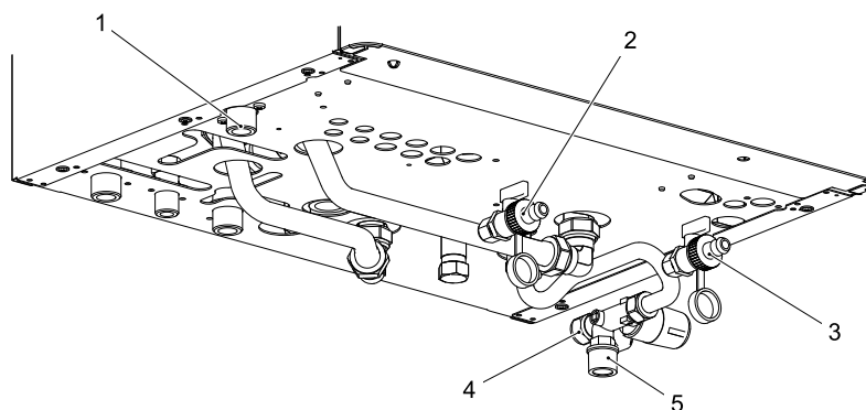
Rys. 9: Dolna część WGB-K
