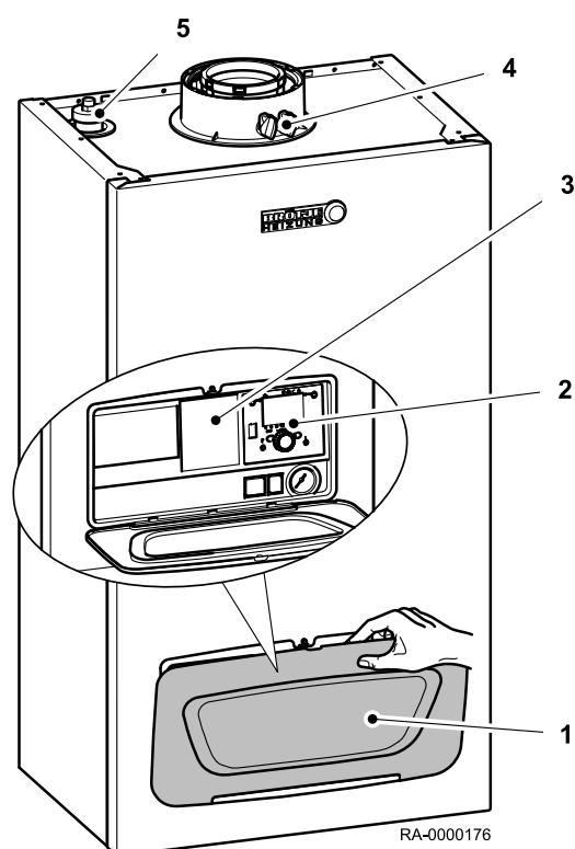
Rys.1 Ogólny widok kotła WGB EVO
