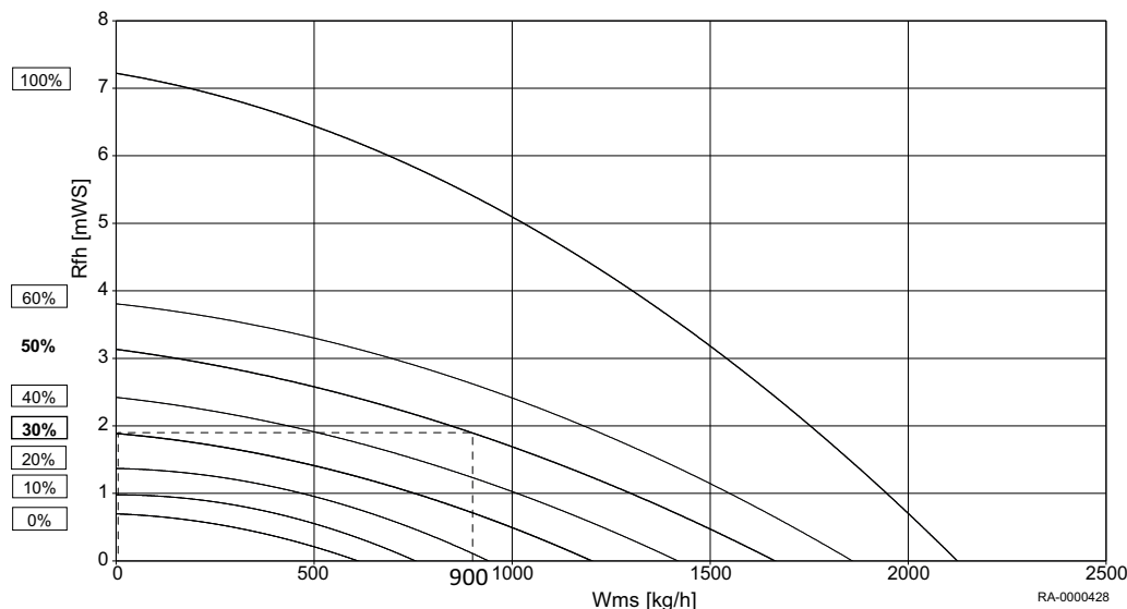
Rys.18 Przykład łącznego ciśnienia dynamicznego
