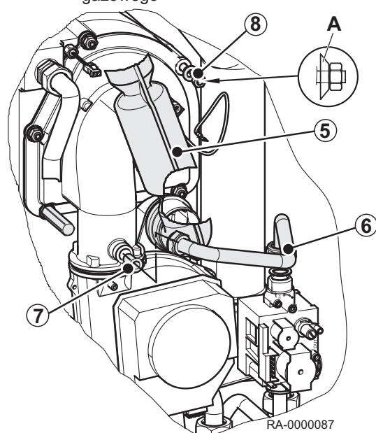
Rys.31 Wymontowywanie palnika gazowego
