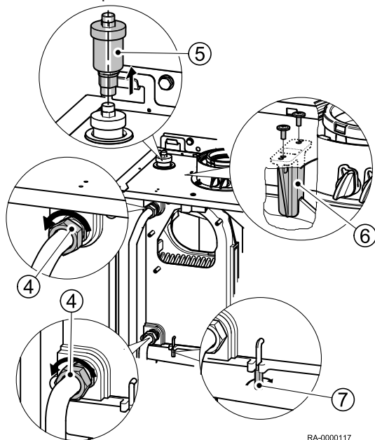
Rys.32 Wymontowywanie wymiennika ciepła
