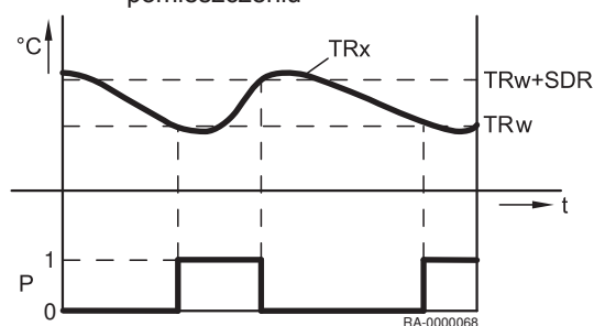
Rys.21 Ograniczenie temperatury w pomieszczeniu
