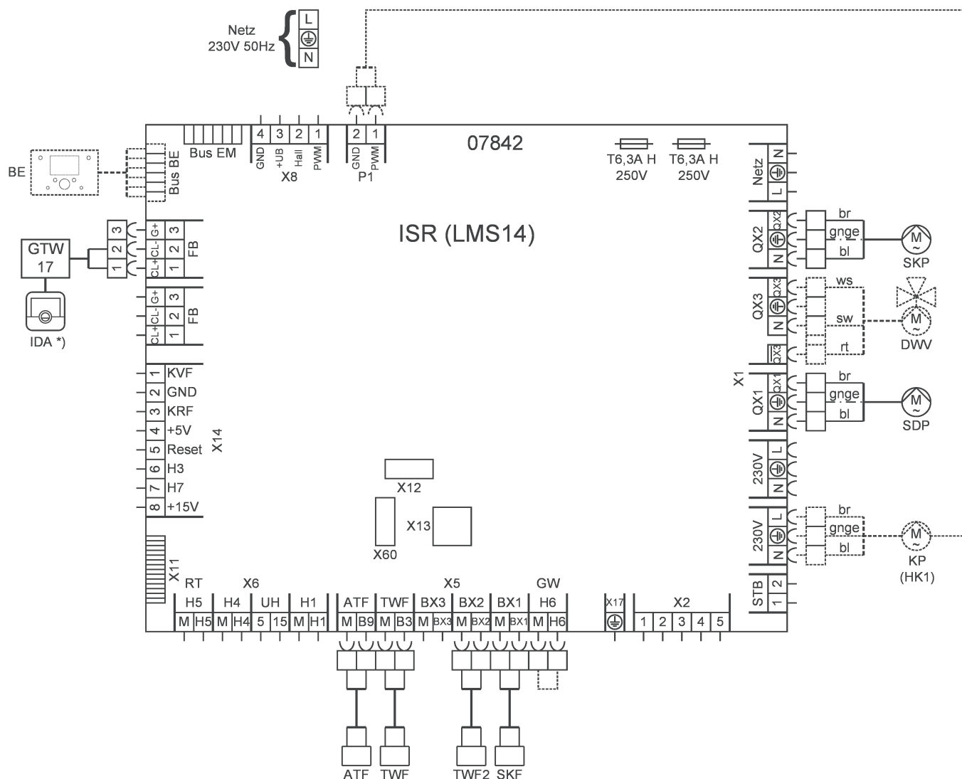
Rys.10 Schemat połączeń elektrycznych
