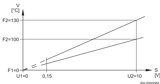
Rys.28 Przykład zapotrzebowania na ciepło 10 V
