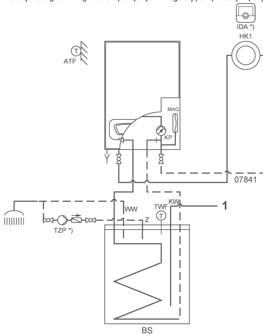
Rys.7 Przykładowa instalacja: obieg c.o. z regulatorem pokojowym i z regulacją temperatury w podgrzewaczu c.w.u.
