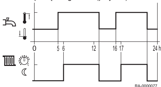
Rys.24 Uruchamianie w zależności od programów sterowania zegarowego pracą obiegów c.o. (przykład)
