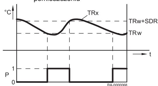
Rys.29 Ograniczenie temperatury w pomieszczeniu
