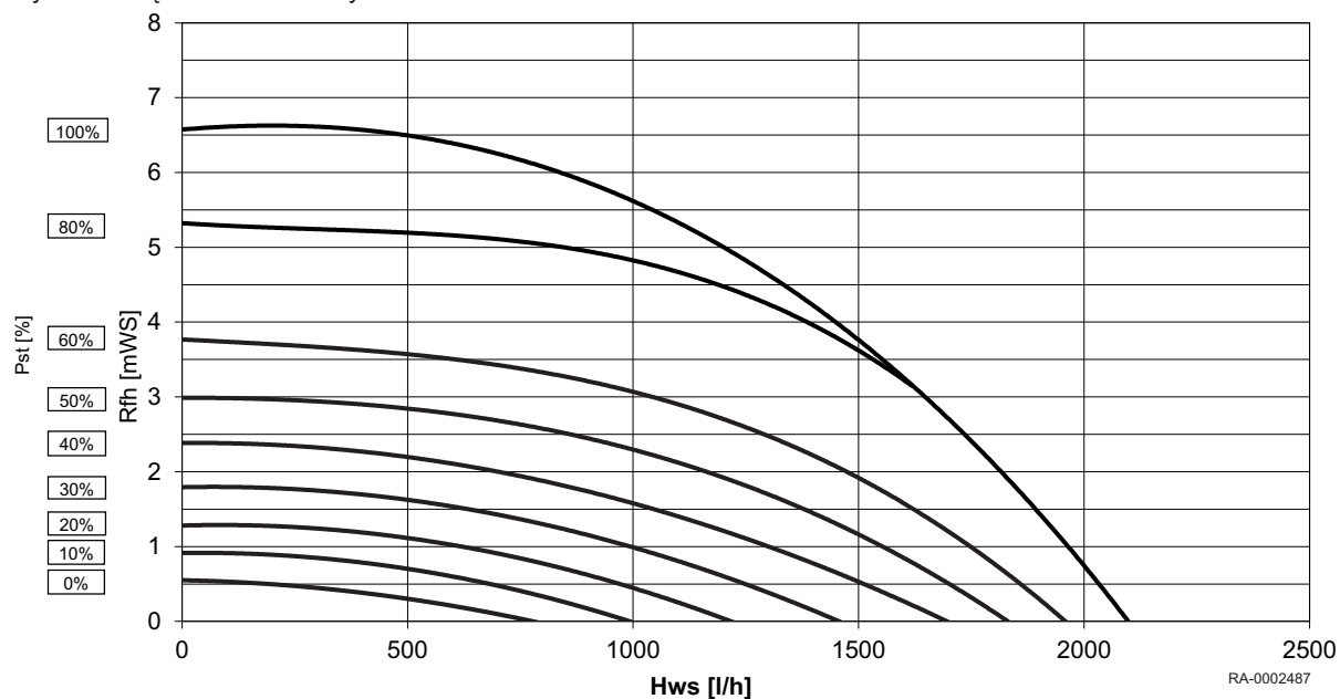
Rys.1 Łączne ciśnienie dynamiczne dla kotła WGB EVO 15 - 20
