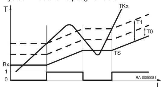
Rys.38 Ładowanie podgrzewacza
