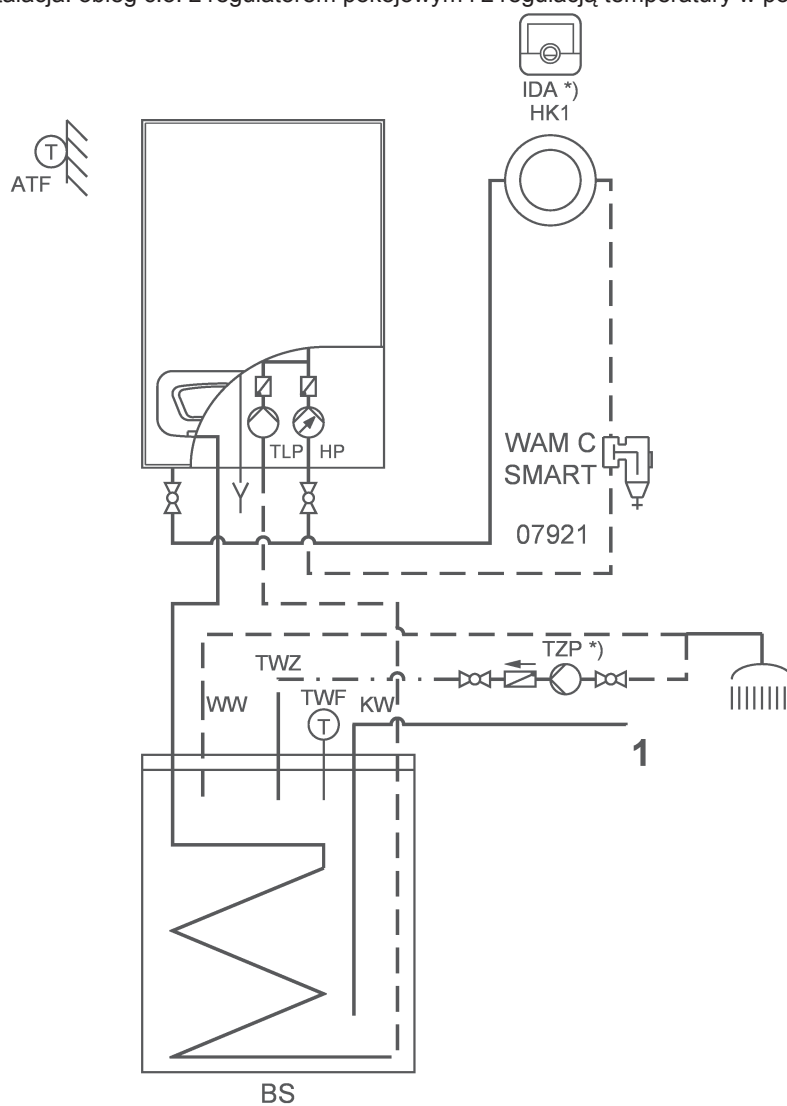
Rys.12 Przykładowa instalacja: obieg c.o. z regulatorem pokojowym i z regulacją temperatury w podgrzewaczu c.w.u.
