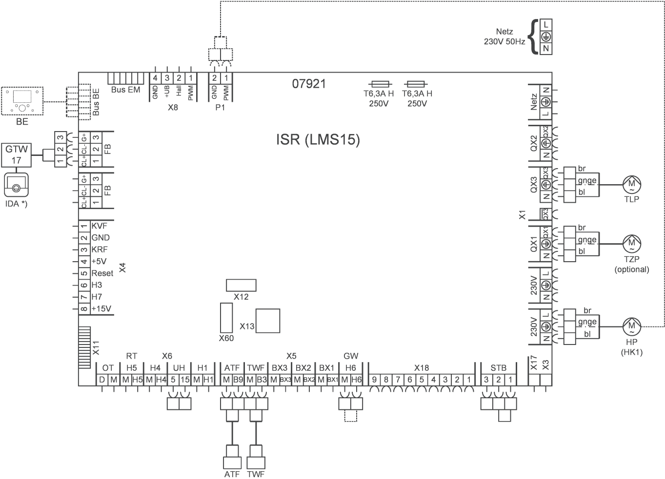
Rys.13 Schemat połączeń elektrycznych
