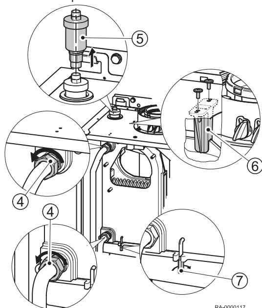
Rys.46 Wymontowywanie wymiennika ciepła
