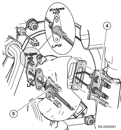
Rys.44 Wymontowywanie elektrody zapłonowej i jonizacyjnej
