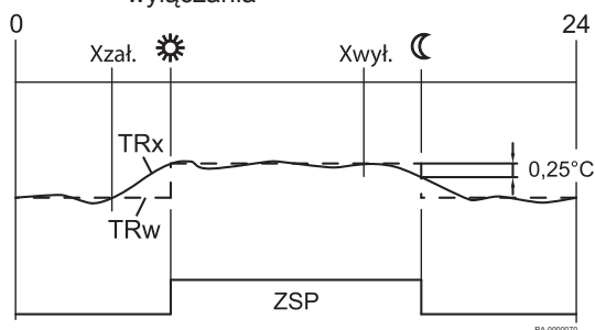
Rys.31 Optymalizacja załączania i wyłączania
