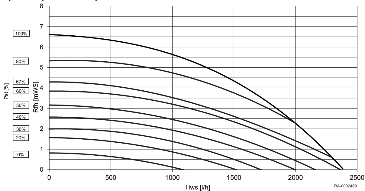
Rys.3 Łączne ciśnienie dynamiczne WGB EVO 38
