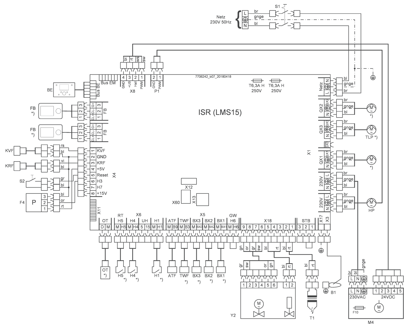
Rys.5 Schemat połączeń elektrycznych WGB EVO 15 - 28
