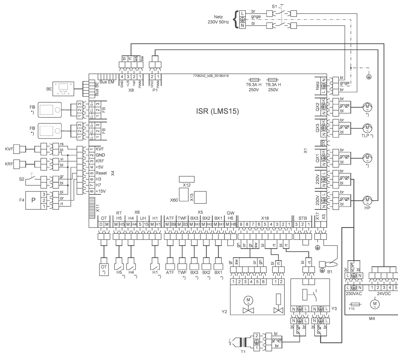
Rys.6 Schemat połączeń elektrycznych WGB EVO 38
