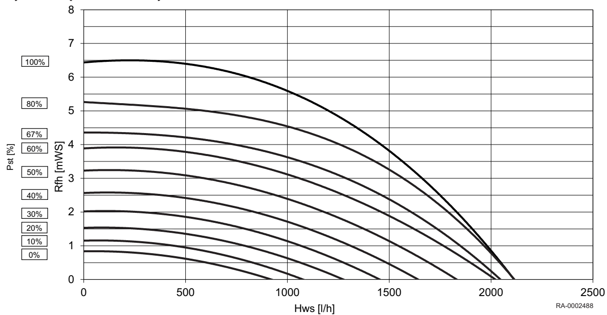
Rys.2 Łączne ciśnienie dynamiczne dla kotła WGB EVO 28
