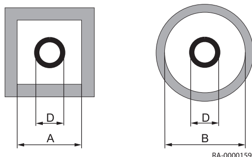
Rys.20 Minimalne wymiary przewodu kominowego
