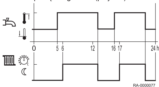
Rys.35 Uruchamianie zgodnie z 4. programem sterowania zegarowego (przykład)
