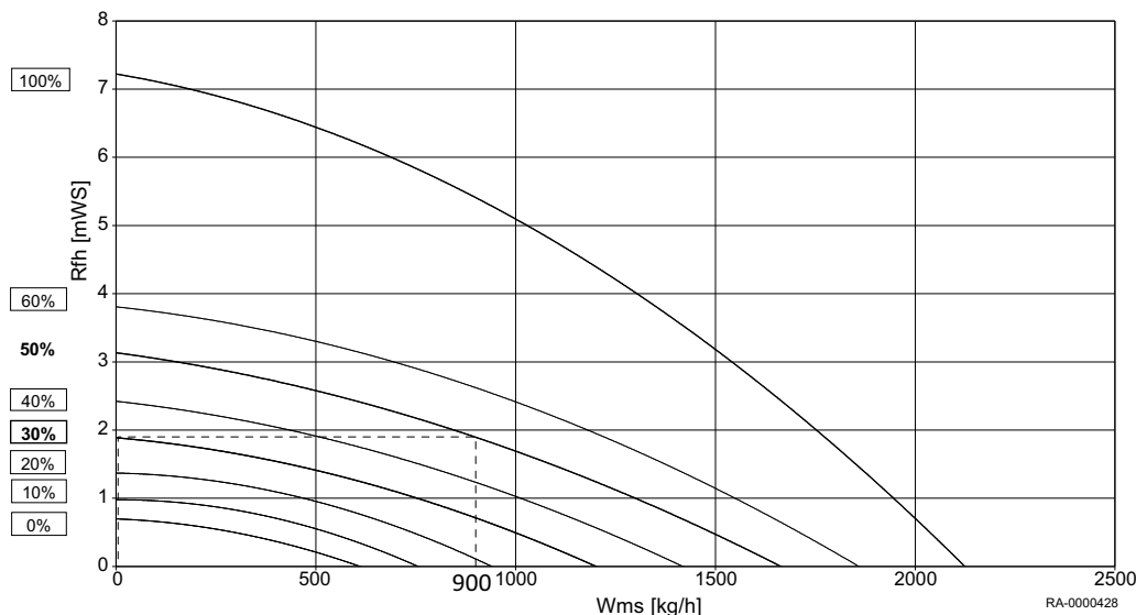
Rys.26 Przykład łącznego ciśnienia dynamicznego
