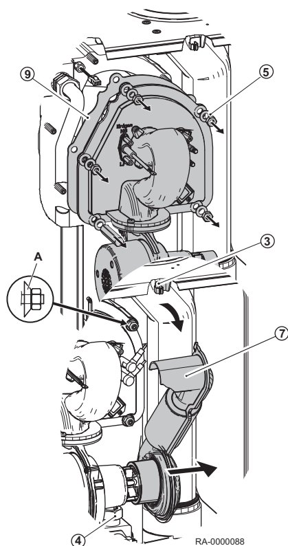
Rys.45 Wymontowywanie palnika gazowego
