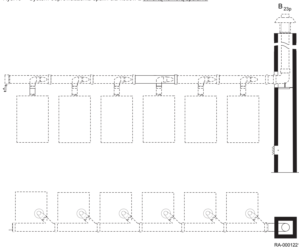
Rys.19 System odprowadzenia spalin dla kotłów z otwartą komorą spalania
