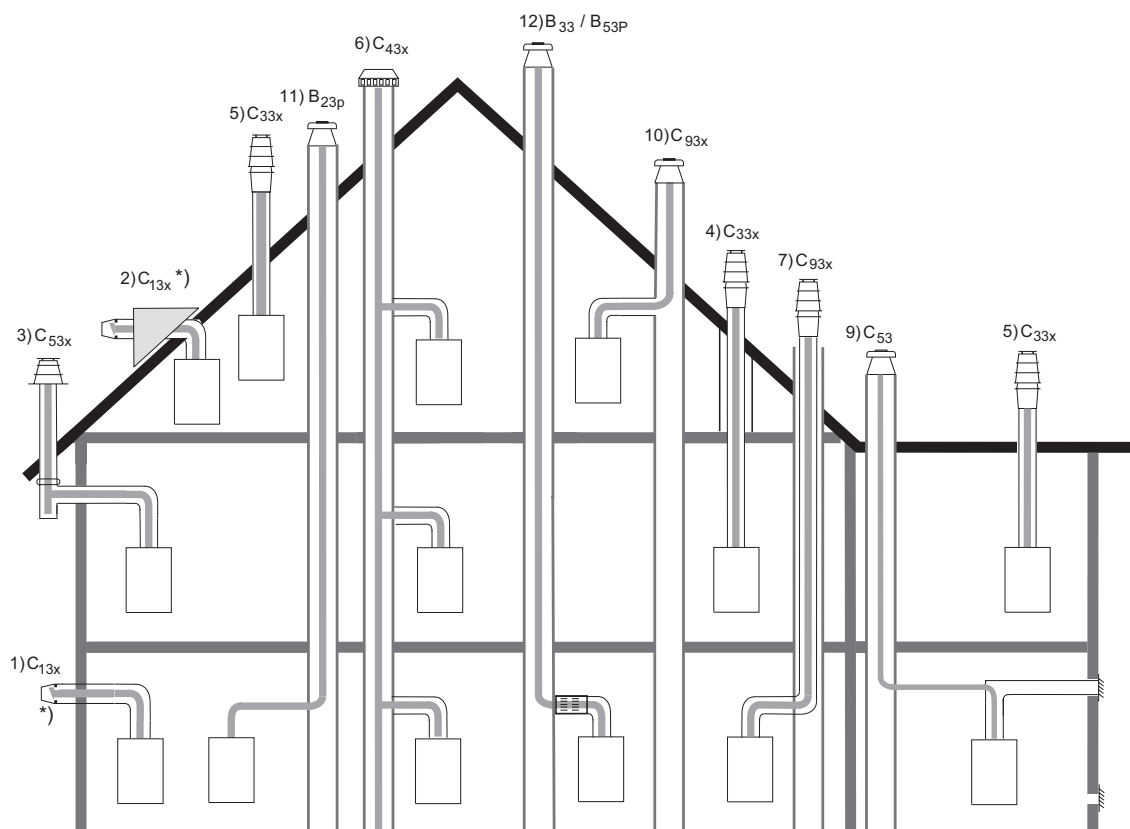
Rys.15 Możliwości zamontowania kotła z zastosowaniem systemu KAS (wyposażenie dodatkowe)
