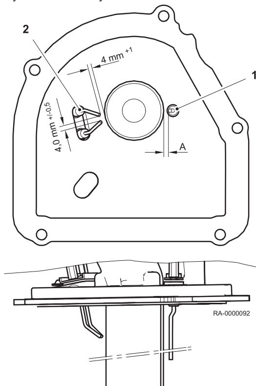
Rys.43 Elektrody
