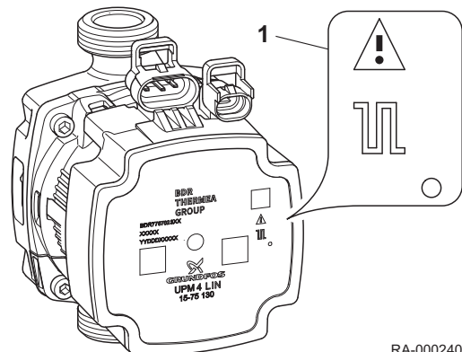
Rys.25 Wyświetlacz stanu pompa obiegowa c.o. UPM4
