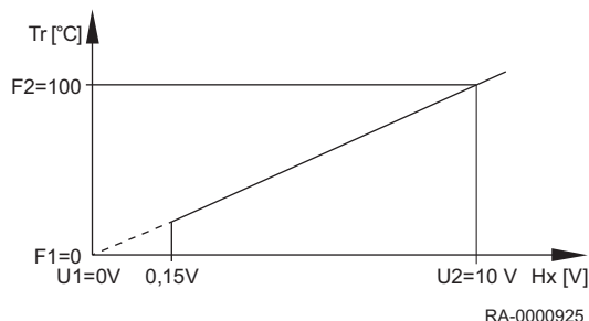
Rys.39 Wartość_napięcia/Wartość_funkcji
