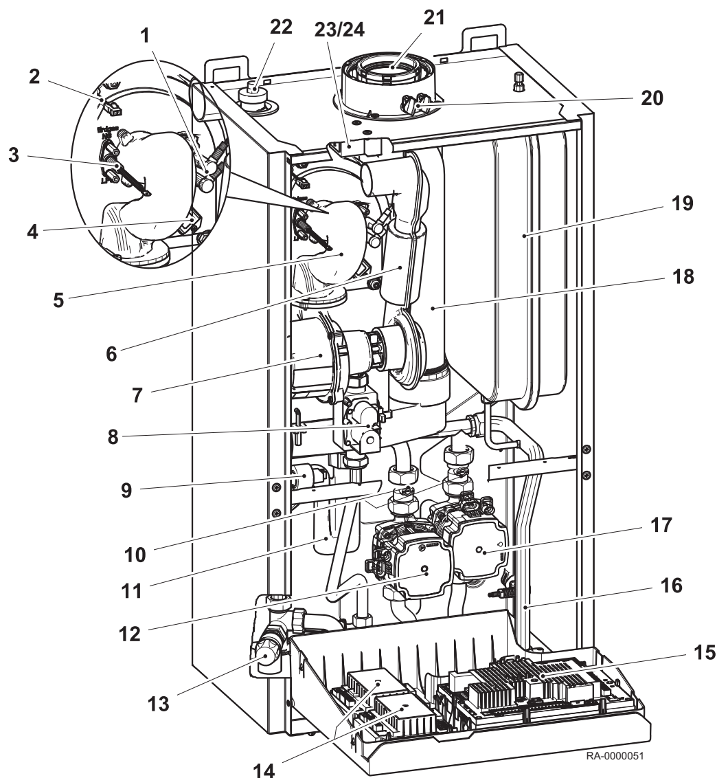
Rys.7 Widok kotła WGB EVO (bez przedniej ścianki i osłony regulatora)
