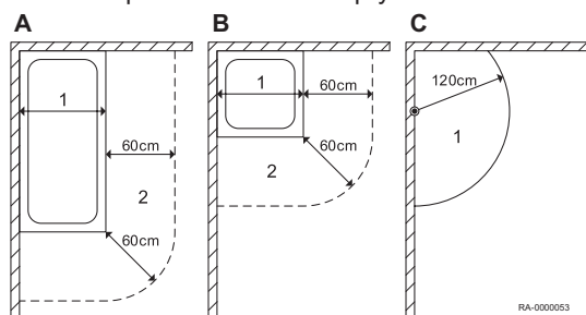
Rys.11 Odległości w łazienkach i pomieszczeniach z prysznicami
