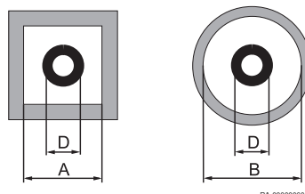
Rys.18 Minimalne wymiary przewodu kominowego
