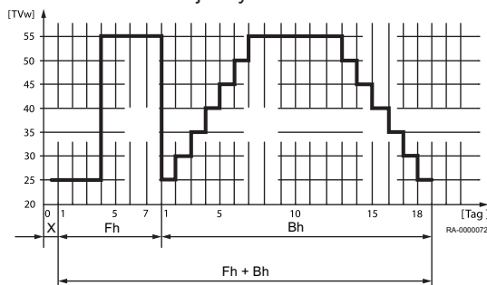
Rys.33 Profil temperaturowy funkcji suszenia jastrychu
