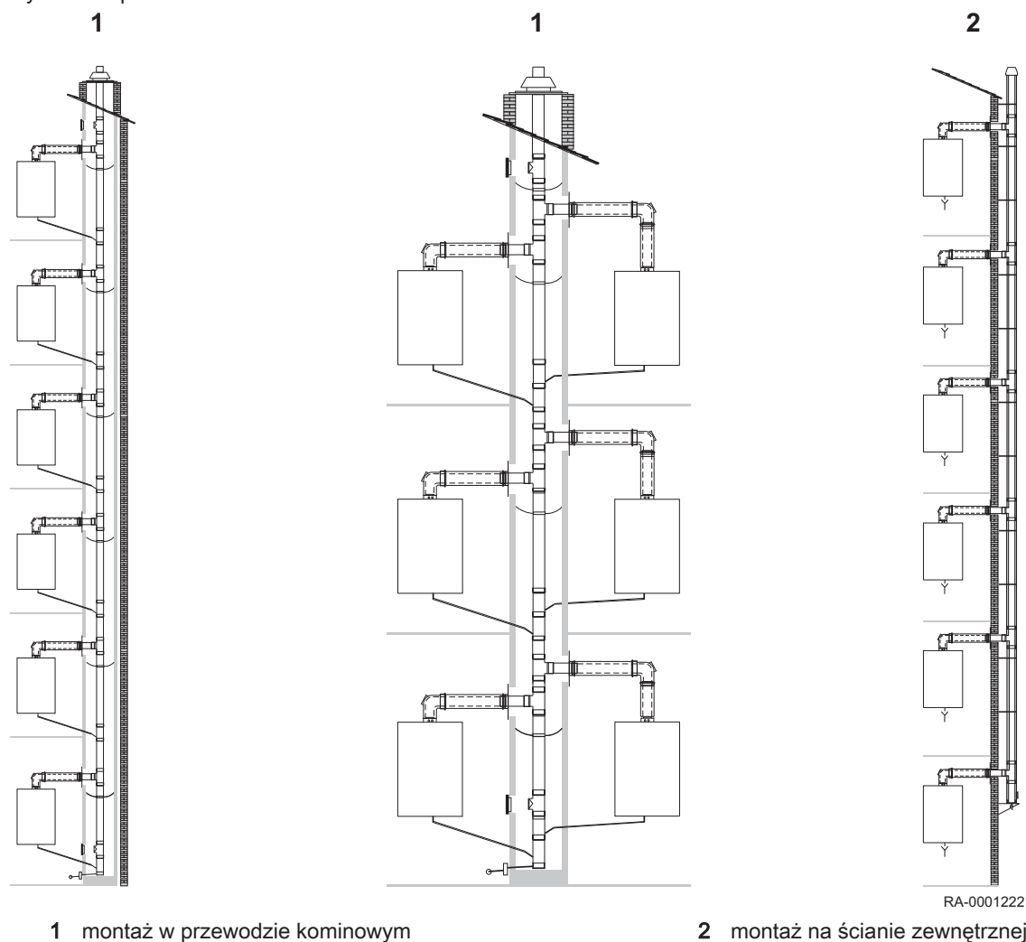
Rys.21 Sposób montażu
