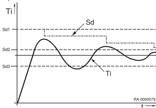
Rys.36 Histereza
