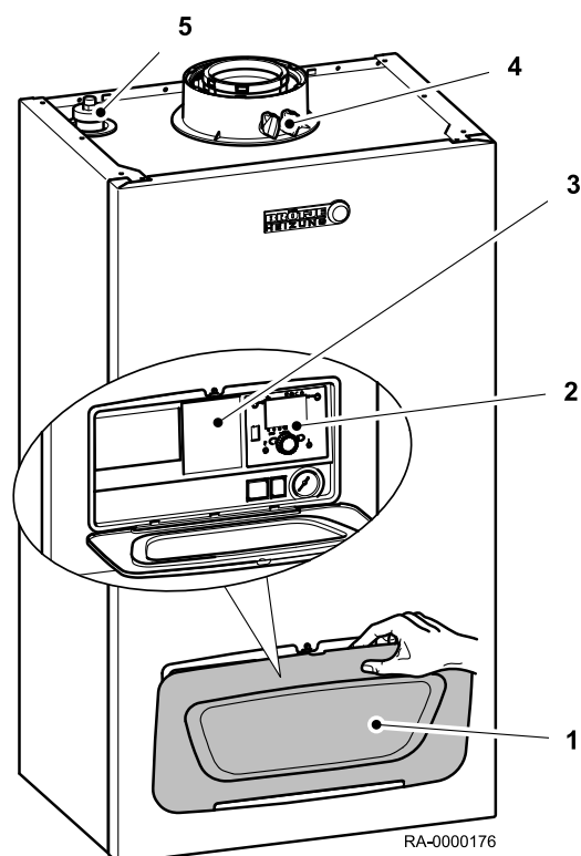
Rys.1 Widok kotła WGB EVO
