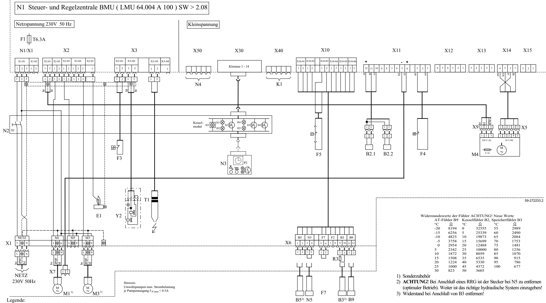
Abb. 3 Schaltplan WGB 2.70
