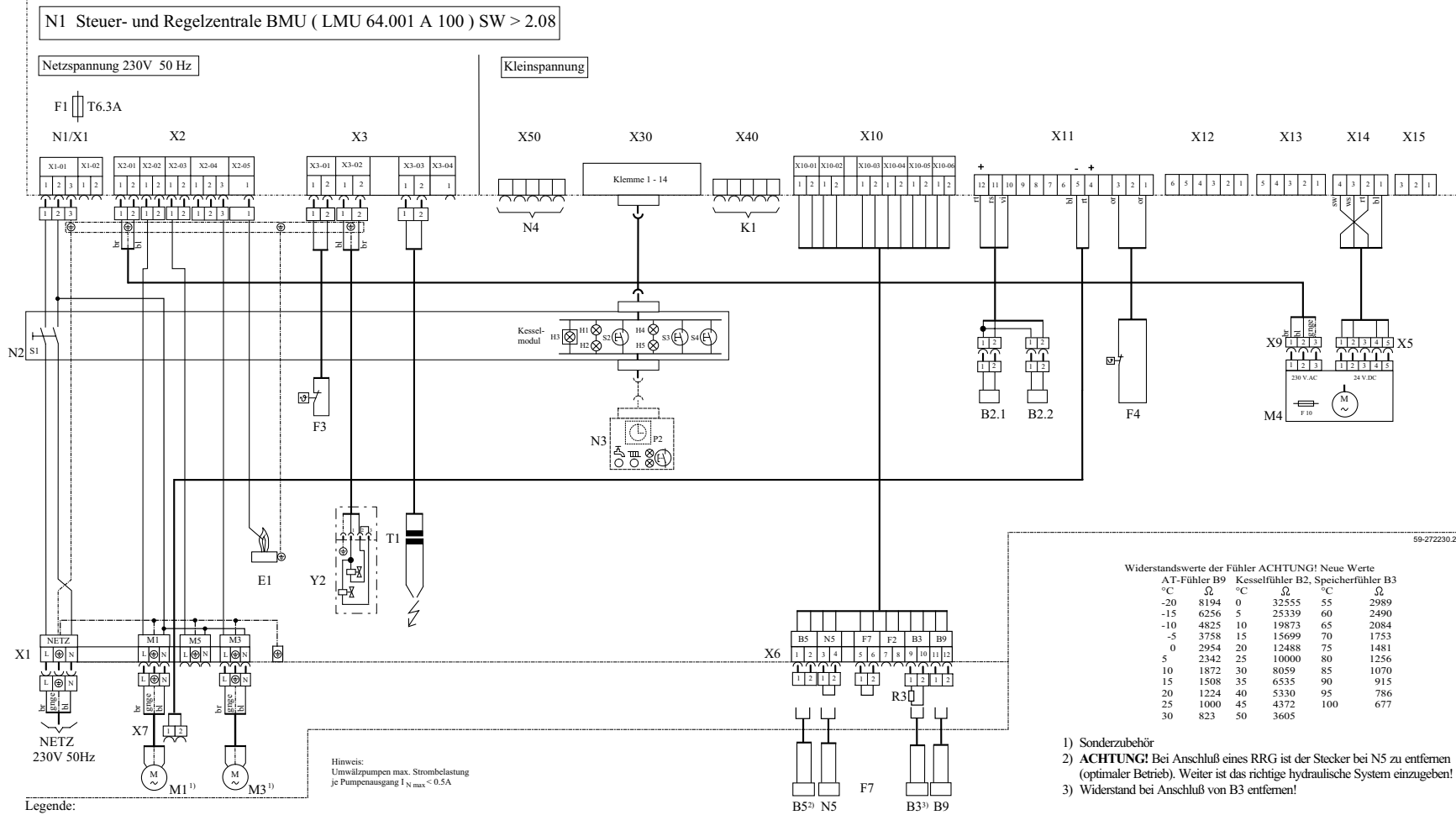
Abb. 2 Schaltplan WGB 2.50
