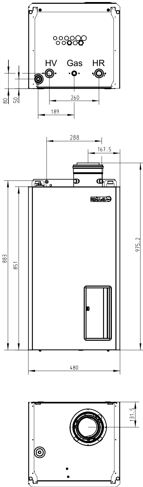
Abb. 1 Abmessungen und Anschlüsse
