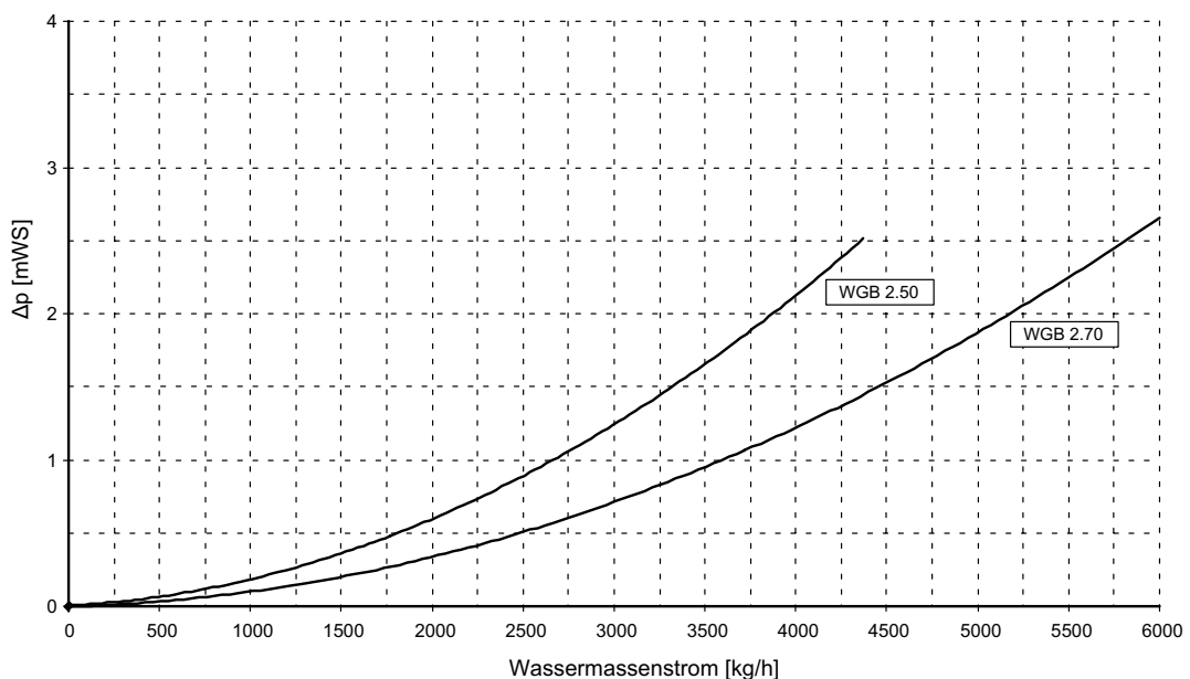
Abb. 5 Hydraulischer Widerstand
