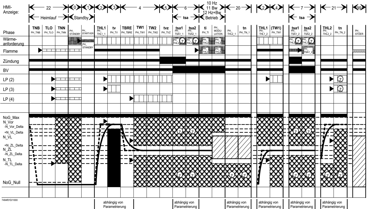
Abb. 16 Programmablauf Steuer- und Regelzentrale BMU (Typ LMU64.001/A100)
