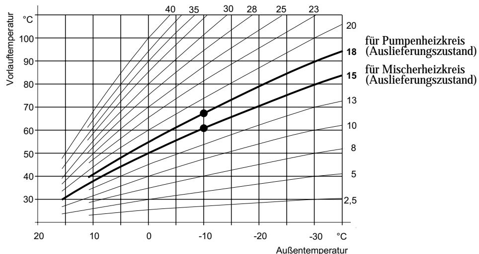
Abb. 9 Heizkennliniendiagramm
